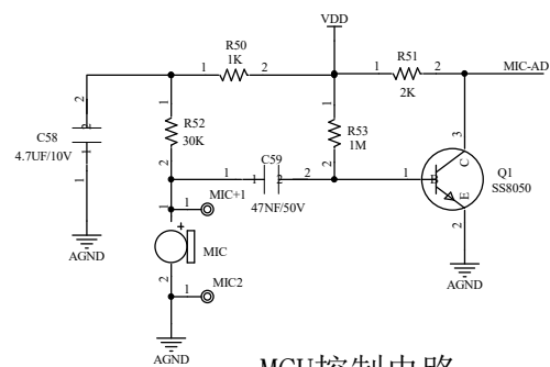
MCU控制电路
