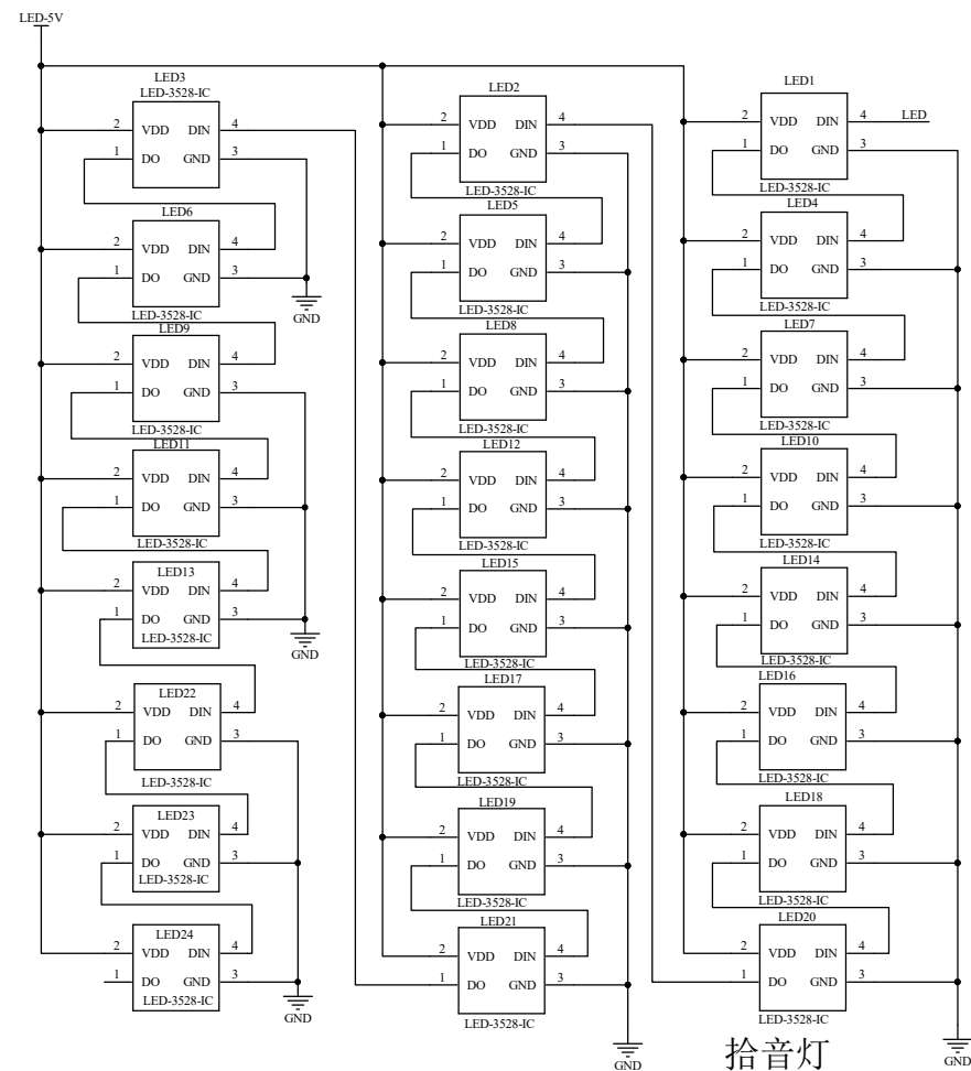
MIC AD输入 幻彩灯控制
