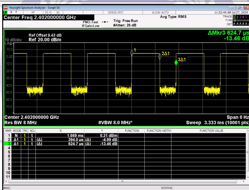
BLE 1M_Channel 0
