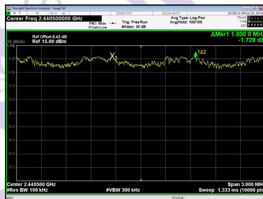
\pi/4 DQPSK
