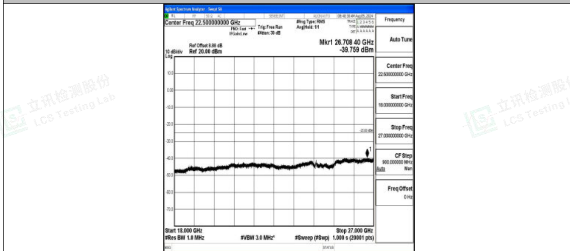
Band7-15MHz-16QAM-20825-1RB#0-18000~27000-PASS
