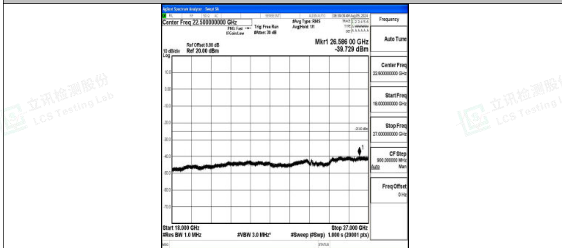
Band7-15MHz-QPSK-20825-1RB#0-18000~27000-PASS
