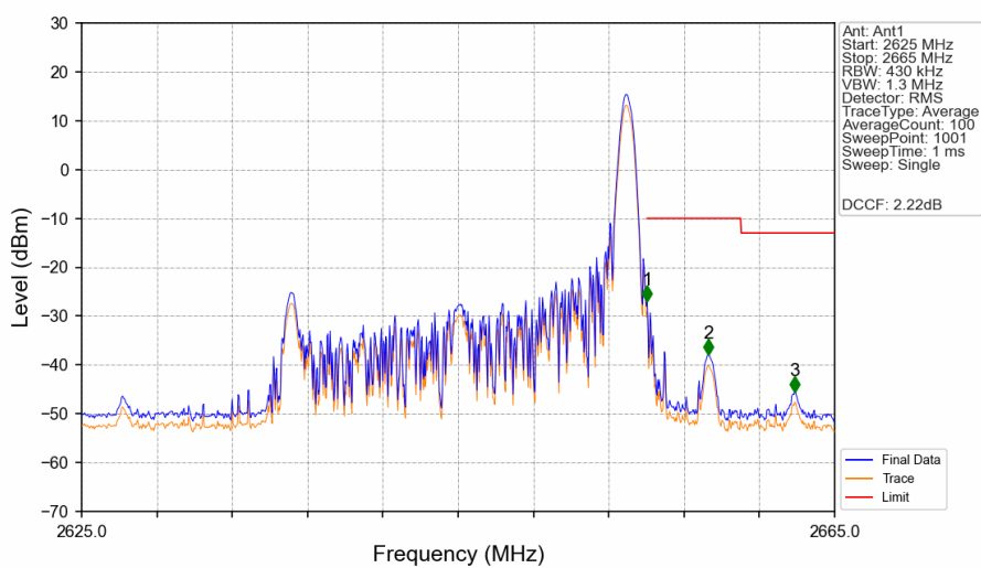
Band41_20MHz_QPSK_HCH_2645MHz_RB_1_99_NTNV
