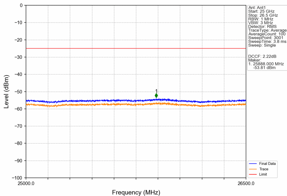
Band41_20MHz_QPSK_HCH_2645MHz_RB_1_99_NTNV
