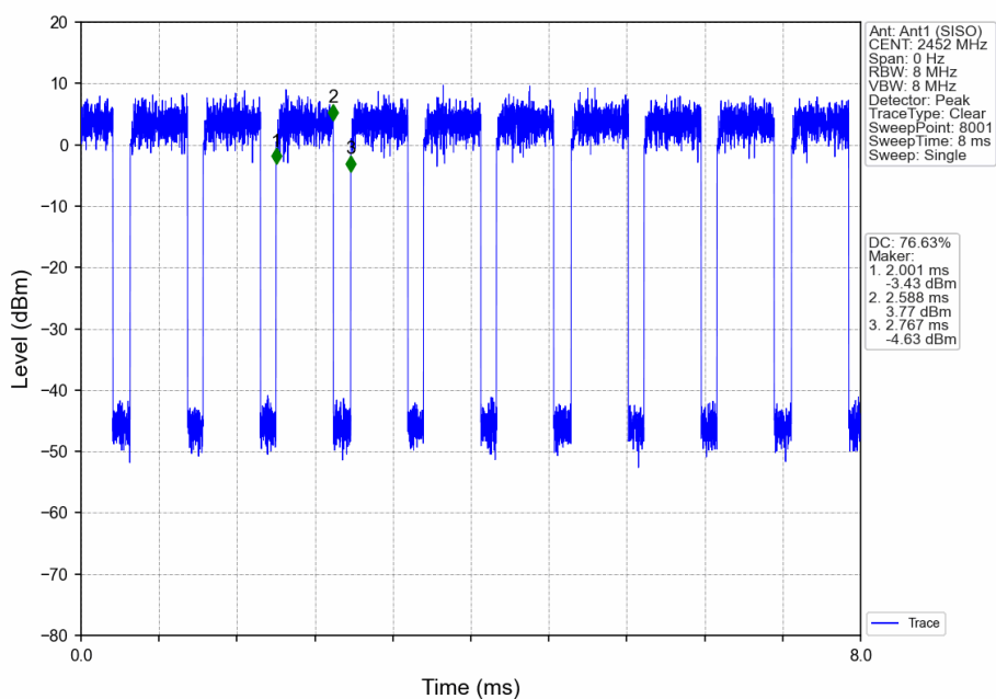
802.11n(HT40)_HCH_2452MHz_Ant1 (SISO)_NTNV
