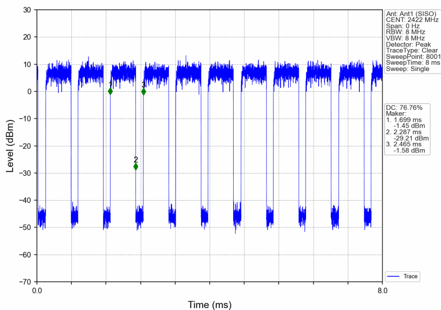
802.11n(HT40)_LCH_2422MHz_Ant1 (SISO)_NTNV
