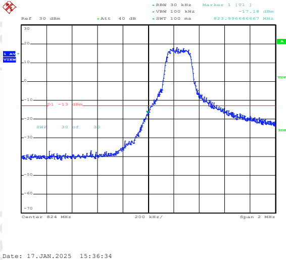
Band5-3MHz-QPSK-20415-1RB#0
