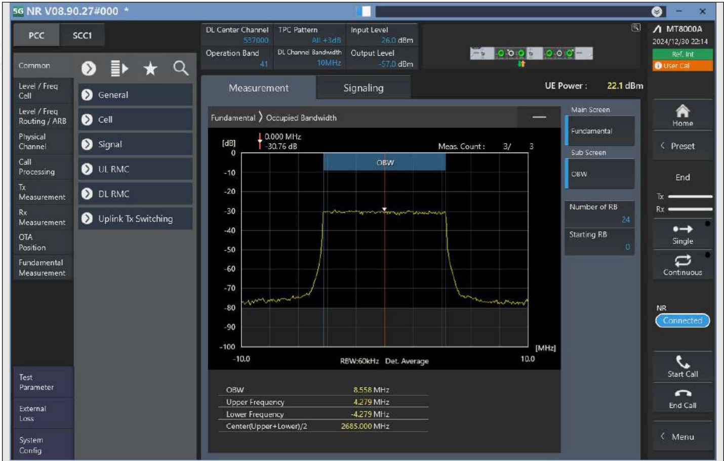
n41_10MHz_30kHz_537000_DFT-s-OFDM QPSK^Outer_Full
