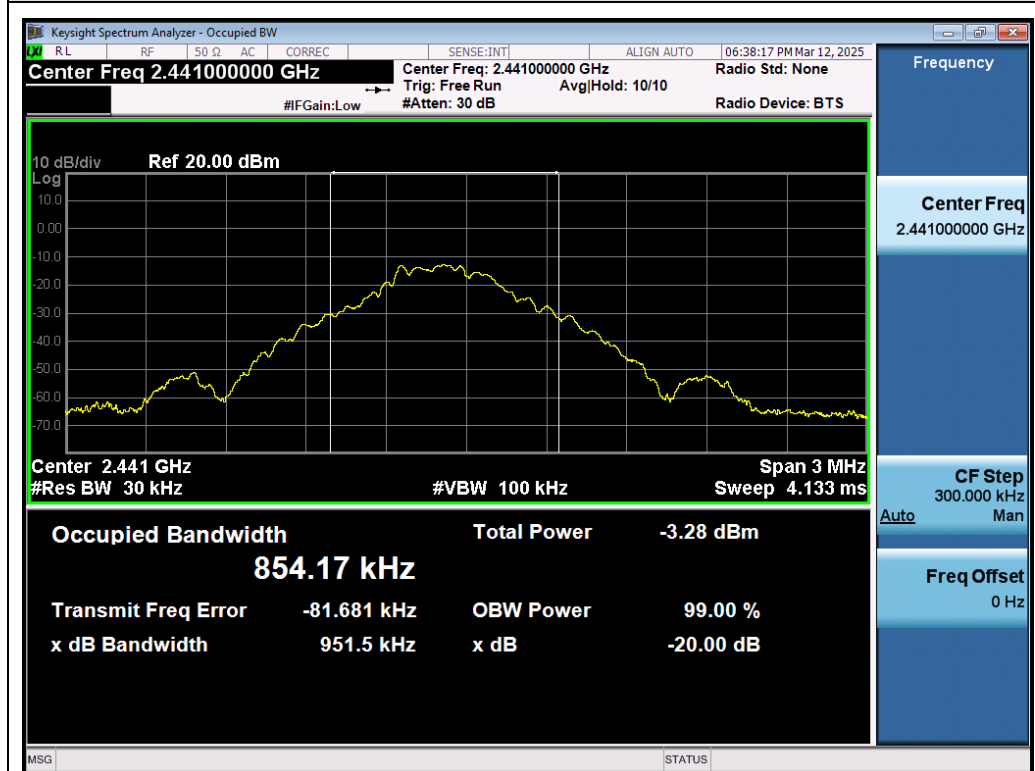
Test_Graph_BR_ANT1_2441_1Mbps_OBW
