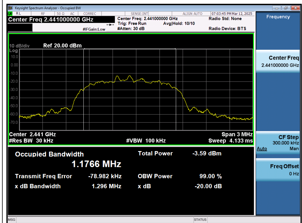
Test_Graph_EDR_ANT1_2441_3Mbps_OBW
