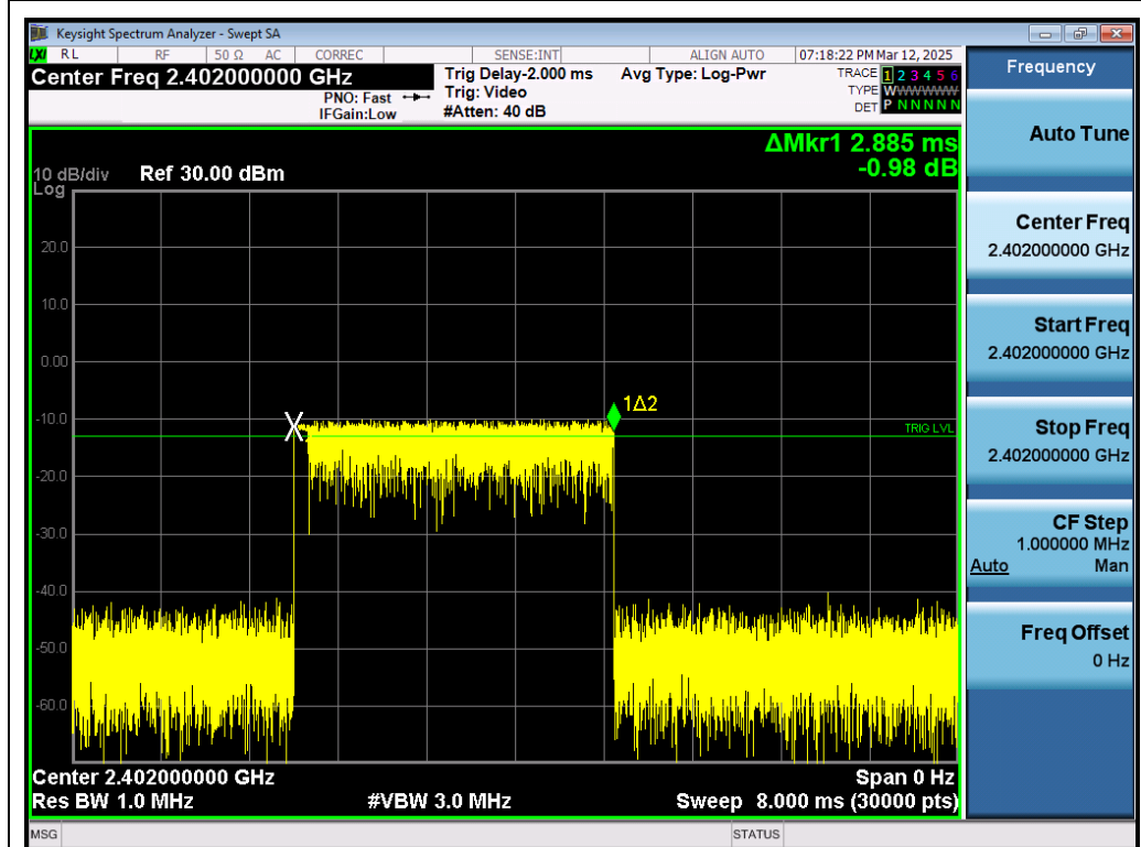
Test_Graph_EDR_HOP_ANT1_NA_3Mbps_2402_Time per Burst
