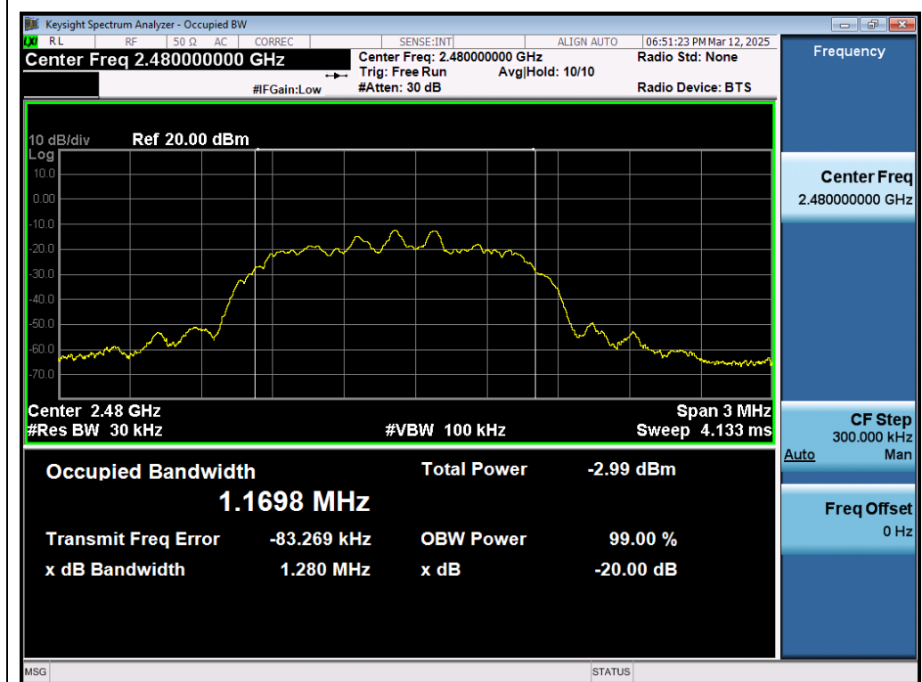
Test_Graph_EDR_ANT1_2480_2Mbps_OBW
