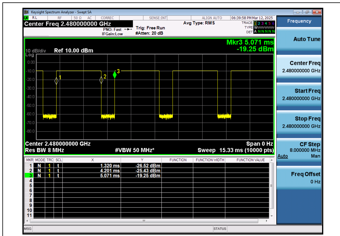
BR-GFSK-ANT1-2480
