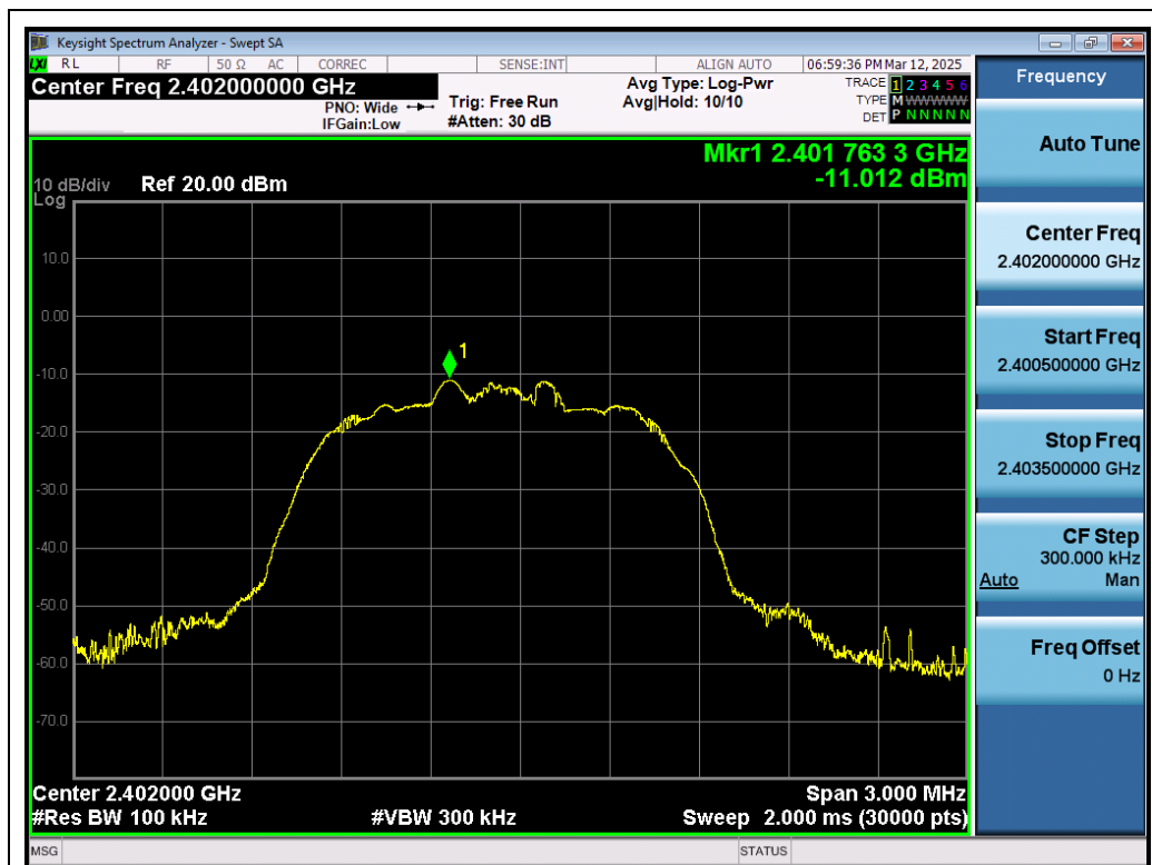
Test_Graph_EDR_ANT1_2402_3Mbps_Reference Level
