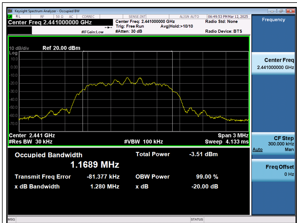
Test_Graph_EDR_ANT1_2441_2Mbps_OBW
