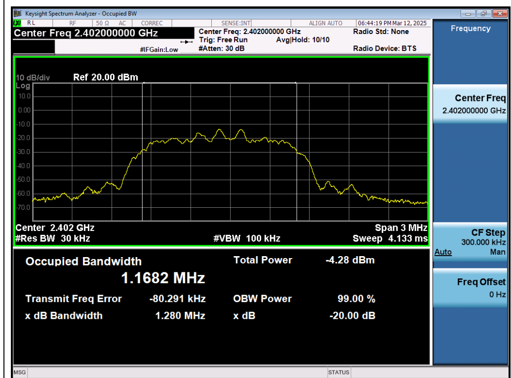
Test_Graph_EDR_ANT1_2402_2Mbps_OBW
