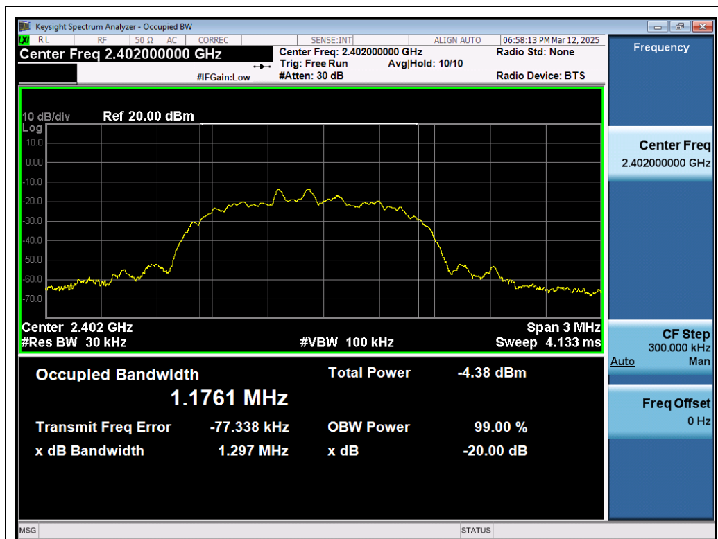
Test_Graph_EDR_ANT1_2402_3Mbps_OBW
