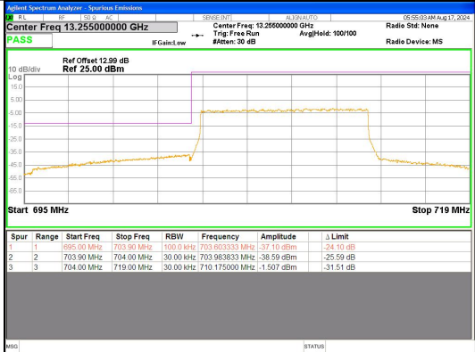
Band 17 10MHz/709.0/Low QPSK 50@0
