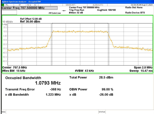
Band 12 1.4MHz/707.5/Mid 16QAM 6@0
