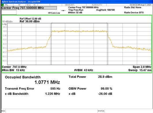
Band 12 1.4MHz/707.5/Mid QPSK 6@0
