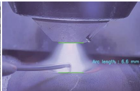
[FIG. 1.1.2] PAW
