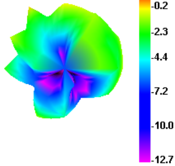
5650.000MHz E1
