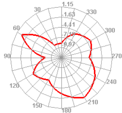
5650.000MHz E2
