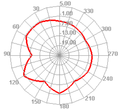
5650.000MHz H
