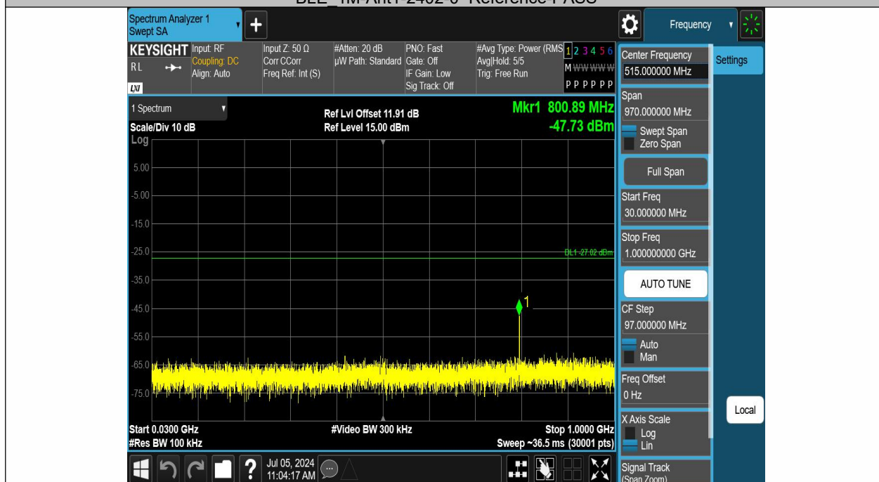
BLE 1M-Ant1-2402-30~1000-PASS
