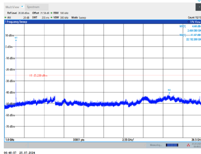
11B_Ant1_2462_1000~26500
