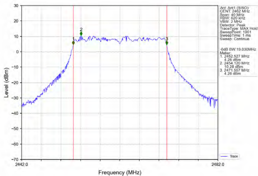
802.11ax(HE20) HCH 2462MHz SU / Ant1 (SISO) NTNV
