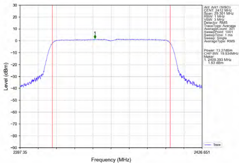
802.11ax(HE20)_LCH_2412MHz_SU / _Ant1 (SISO)_NTNV
