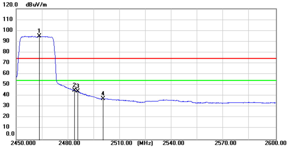
11(HE20)_TX_CH_11_Horizontal_Average
