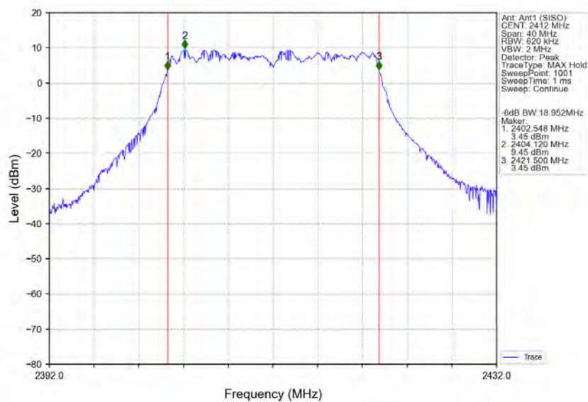
802.11ax(HE20) LCH 2412MHz SU / Ant1 (SISO) NTN
