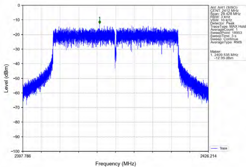
802.11ax(HE20)_LCH_2412MHz_SU_/_Ant1 (SISO)_NTNV
