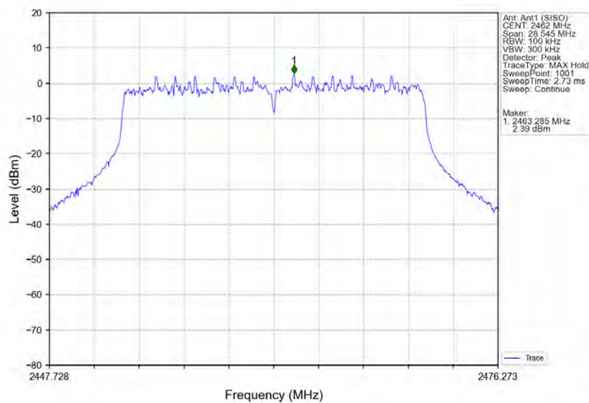
802.11ax(HE20) HCH_2462MHz_SU_ / Ant1 (SISO) NTN
