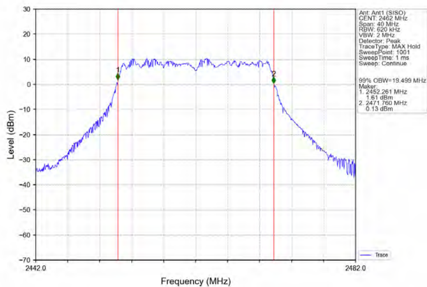
802.11ax(HE20) HCH_2462MHz_SU_ / Ant1 (SISO) NTN
