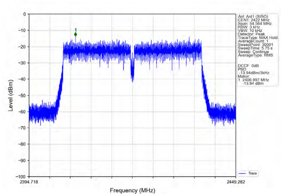
802.11n(HT40) LCH 2422MHz Ant1 (SISO) NTN
