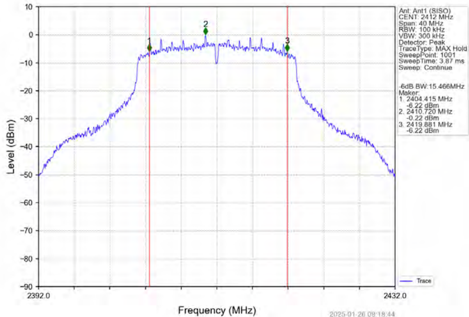
802.11ax(HE20) LCH_2412MHz_RU242_Left_Ant1 (SISO)_NTNV
