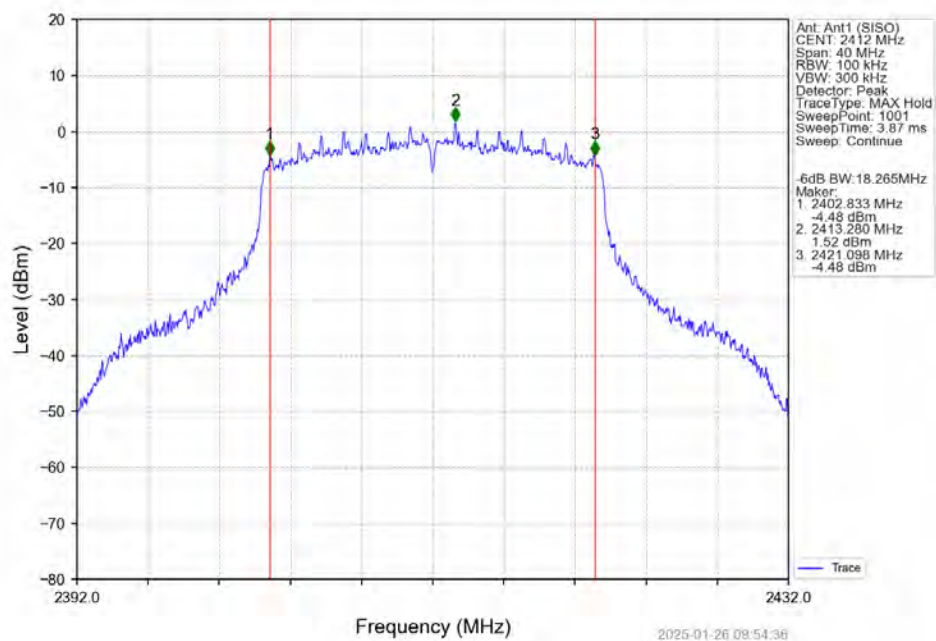
802.11ax(HE20) LCH_2412MHz_RU242_Left_Ant1 (SISO)_NTNV
