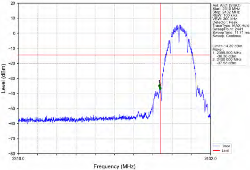
802.11b_LCH_2412MHz_Ant1 (SISO)_NTNV
