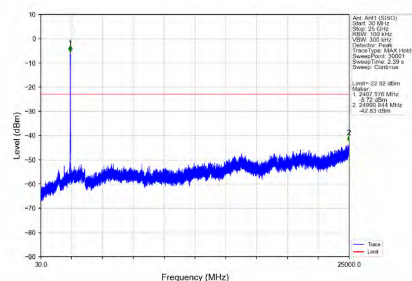
802.11ax(HE20) LCH 2412MHz RU242 Left Ant1 (SISO) NTN
