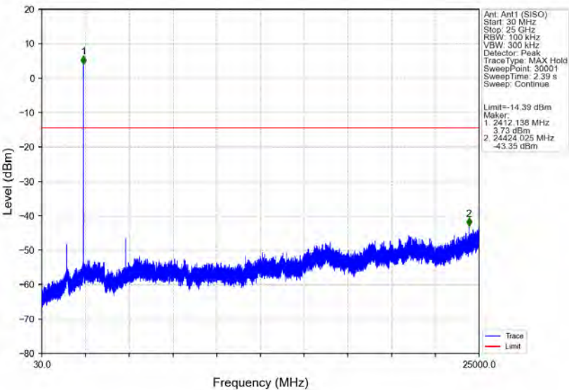
802.11b_LCH_2412MHz_Ant1 (SISO)_NTNV
