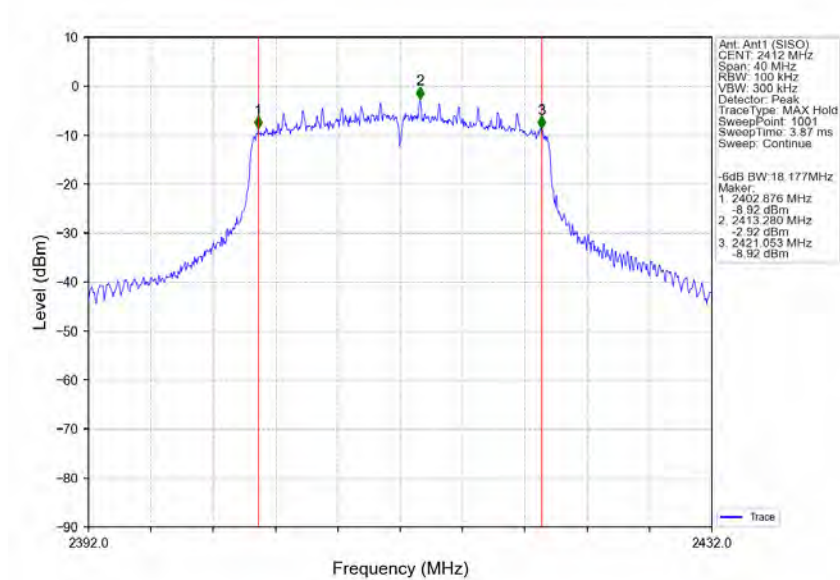
802.11ax(HE20) LCH 2412MHz RU242 Left Ant1 (SISO) NTNv
