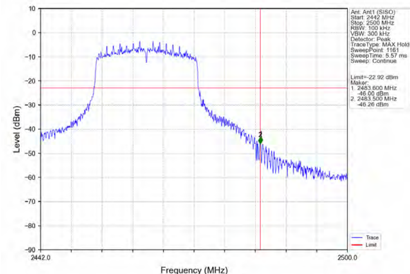
802.11ax(HE20) HCH 2462MHz RU242 Left Ant1 (SISO) NTNv
