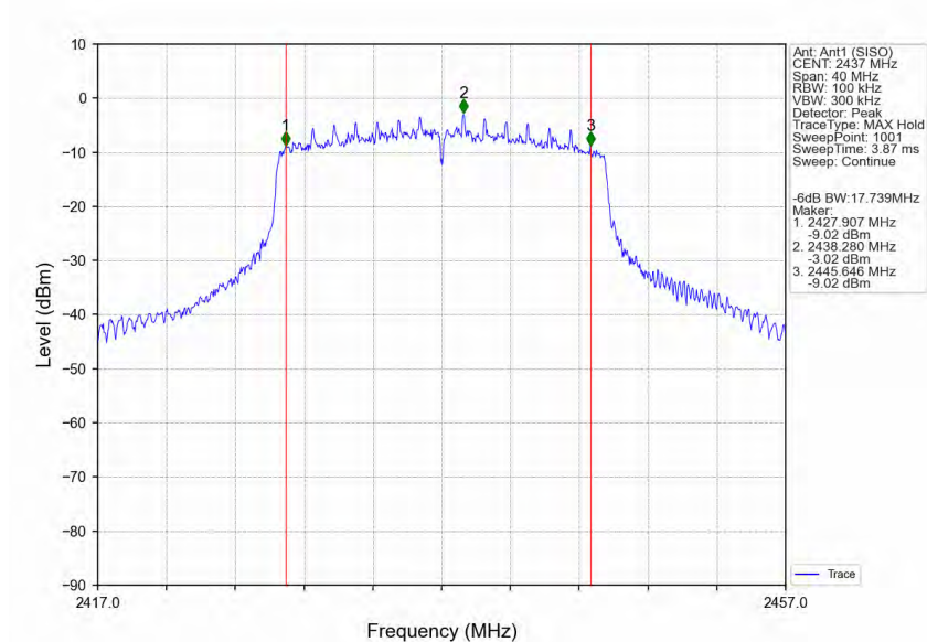
802.11ax(HE20) MCH 2437MHz RU242 Left Ant1 (SISO) NTNv
