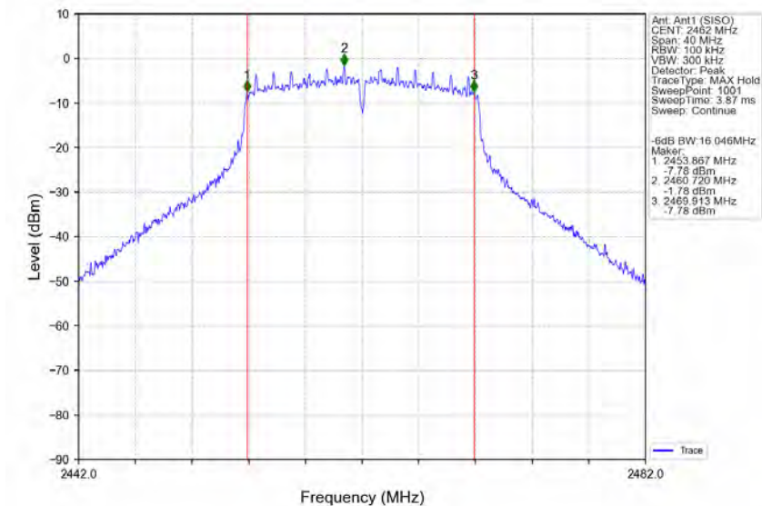
802.11g_HCH_2462MHz_Ant1 (SISO)_NTNV
