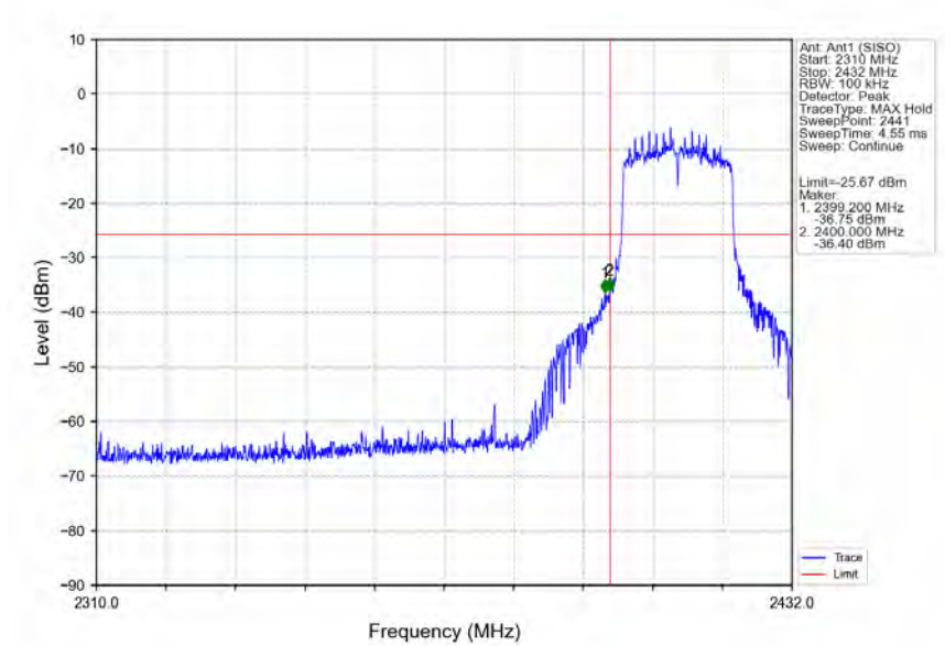
802.11ax(HEW20) LCH 2412MHz RU242 Left Ant1 (SISO) NTNv
