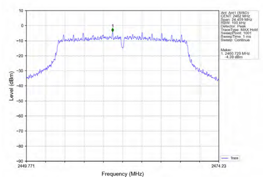
802.11g_HCH_2462MHz_Ant1 (SISO)_NTNV
