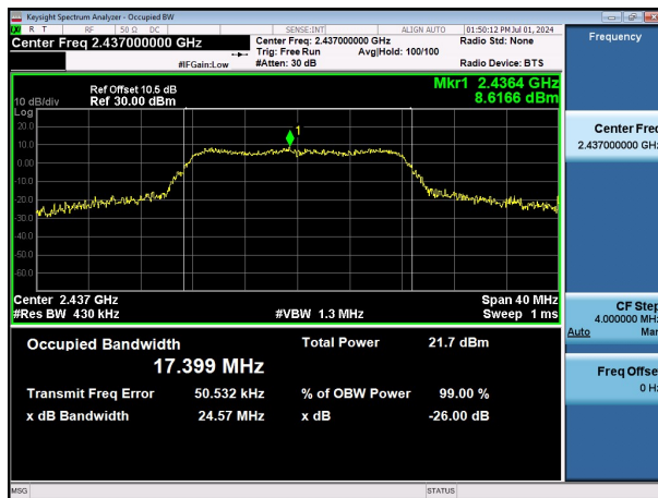
11G-Ant1-2437
