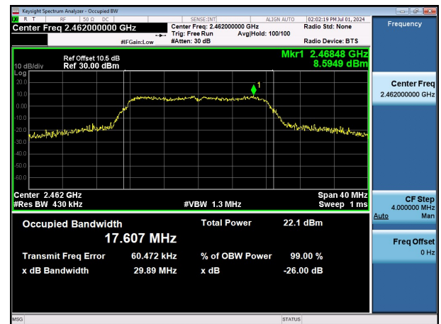
11G-Ant1-2462
