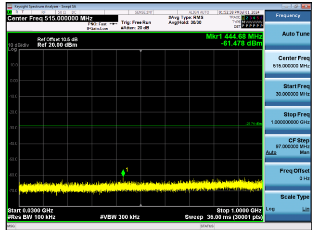
11G-Ant1-2437-30~1000-PASS
