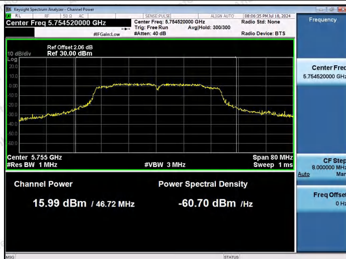
11N40SISO-Ant1-5755-PASS
