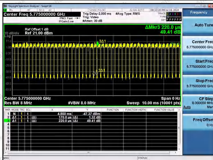
NTNV-11AC80SISO-Ant1-5775
