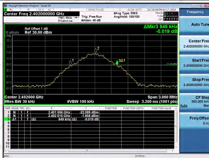
DH5-Ant1-2402
