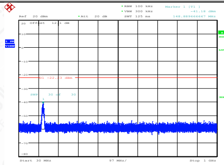
11G-Ant1-2462-30~1000-PASS
