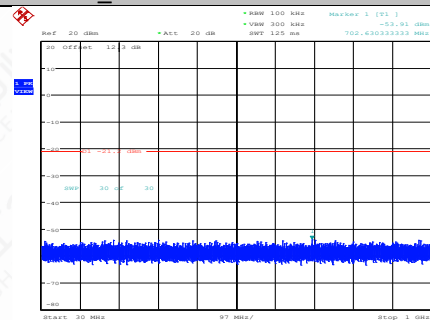
BLE_500K-Ant1-2440-30~1000-PASS
