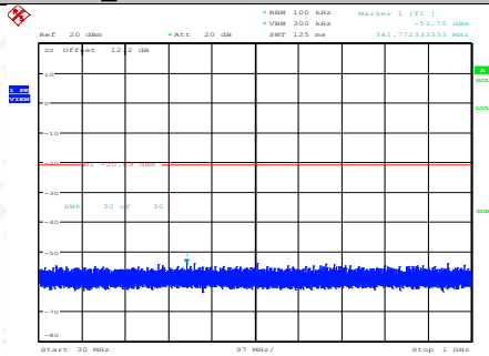
BLE_500K-Ant1-2402-30~1000-PASS
