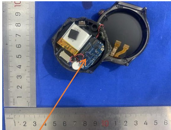
Antenna
