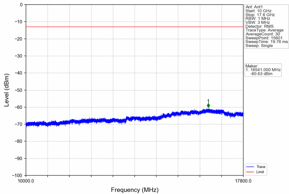
Band66 1.4MHz QPSK LCH 1710.7MHz RB 6 0 NTV
