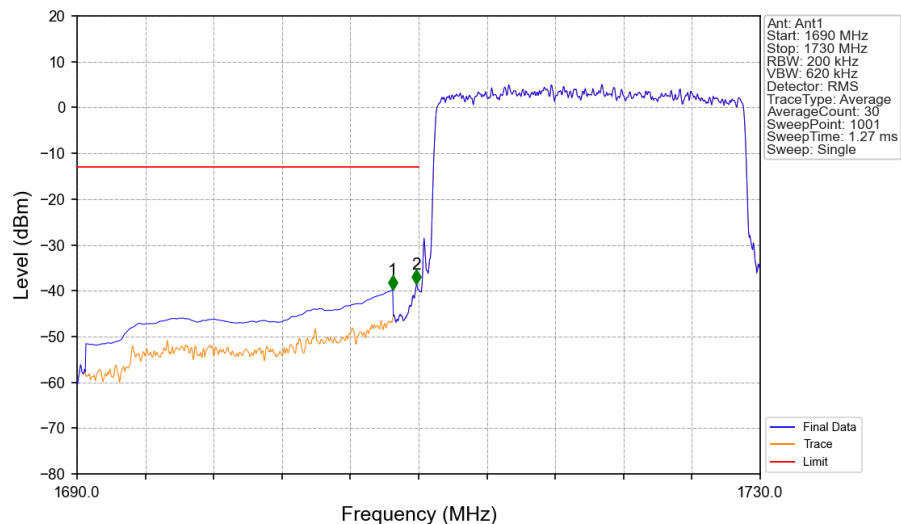
Band4 20MHz QPSK LCH 1720MHz RB 100 0 NTNV
