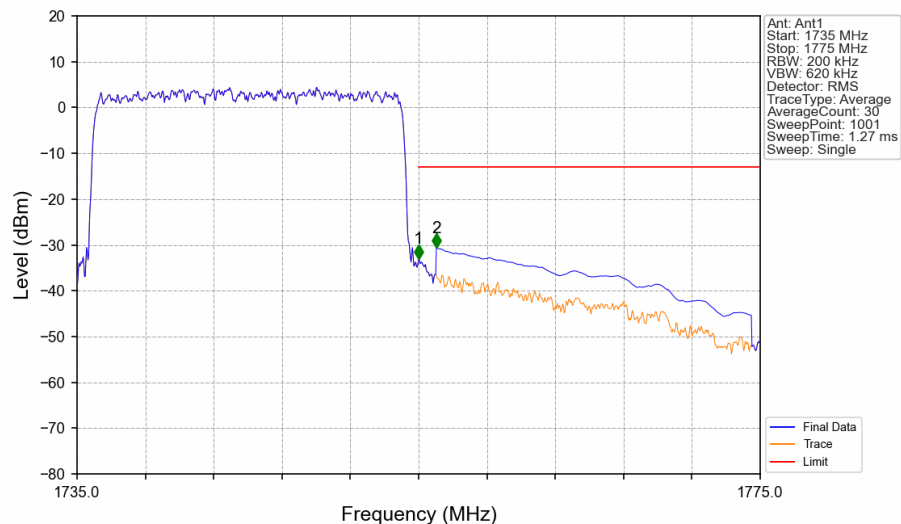
Band4 20MHz QPSK HCH 1745MHz RB 100 0 NTNV
