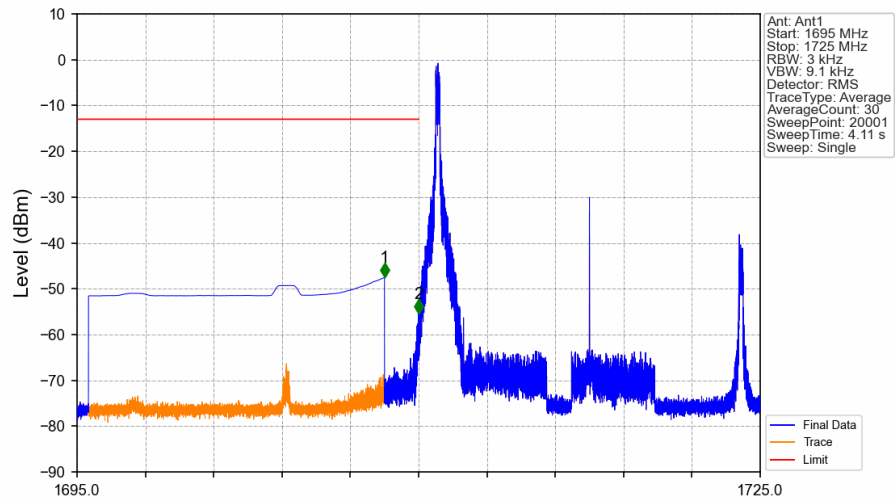
Band4_15MHz_QPSK_LCH_1717.5MHz_RB_1_0_NTNV
