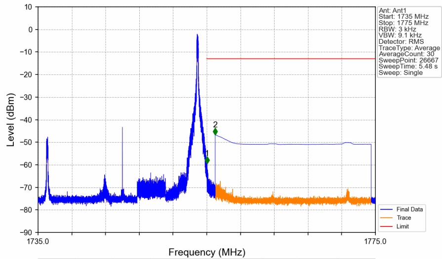
Band4 20MHz QPSK HCH 1745MHz RB 1 99 NTNV
