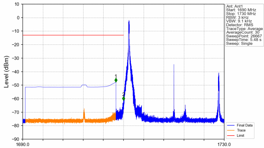
Band4_20MHz_QPSK_LCH_1720MHz_RB_1_0_NTNV
