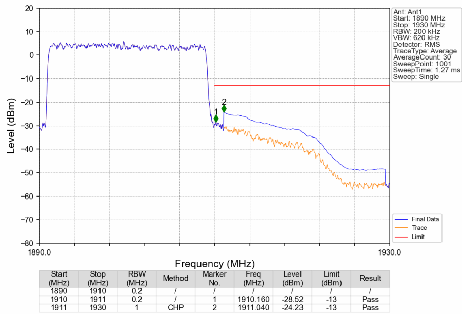
Band2 20MHz QPSK HCH 1900MHz RB 100 0 NTNV
