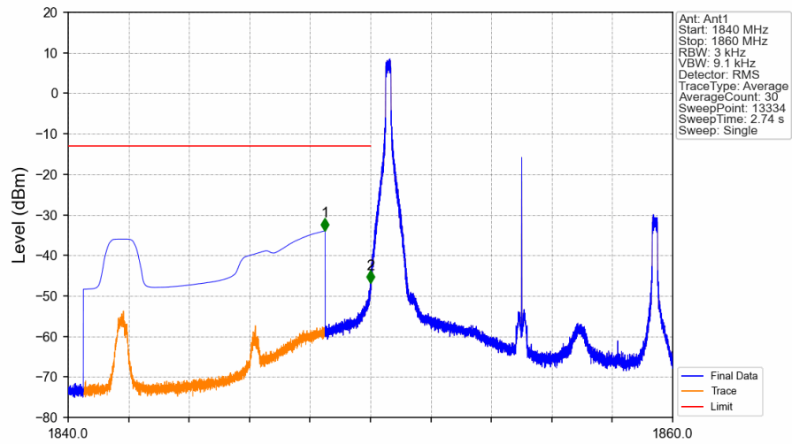
Band2_10MHz_QPSK_LCH_1855MHz_RB_1_0_NTNV
