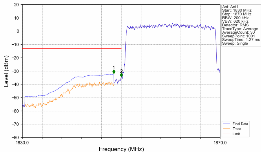
Band2_20MHz_QPSK_LCH_1860MHz_RB_100_0_NTNV
