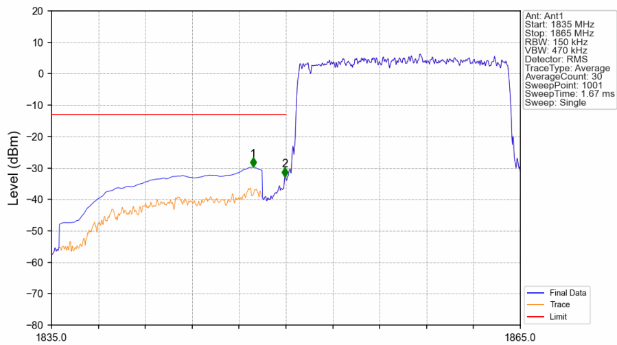
Band2 15MHz QPSK LCH 1857.5MHz RB 75 0 NTNV
