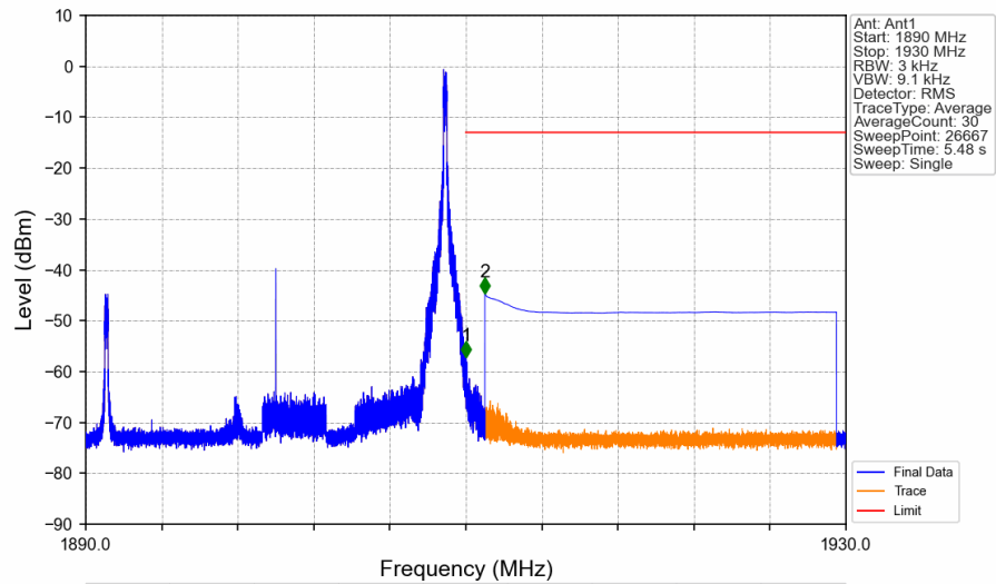
Band2 20MHz QPSK HCH 1900MHz RB 1 99 NTNV
