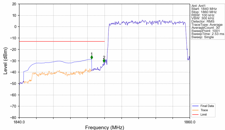
Band2_10MHz_QPSK_LCH_1855MHz_RB_50_0_NTNV
