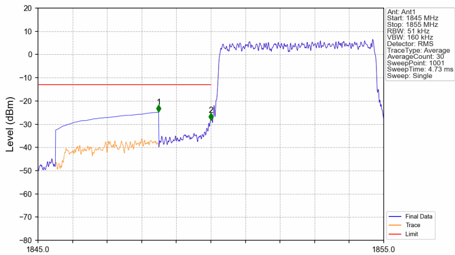
Band2 5MHz QPSK LCH 1852.5MHz RB 25 0 NTN
