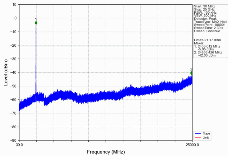
802.11n(HT40)_MCH_2437MHz_Ant1 (SISO)_NTNV
