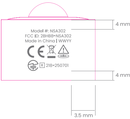
Bottom
