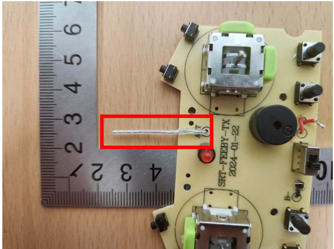
Antenna
