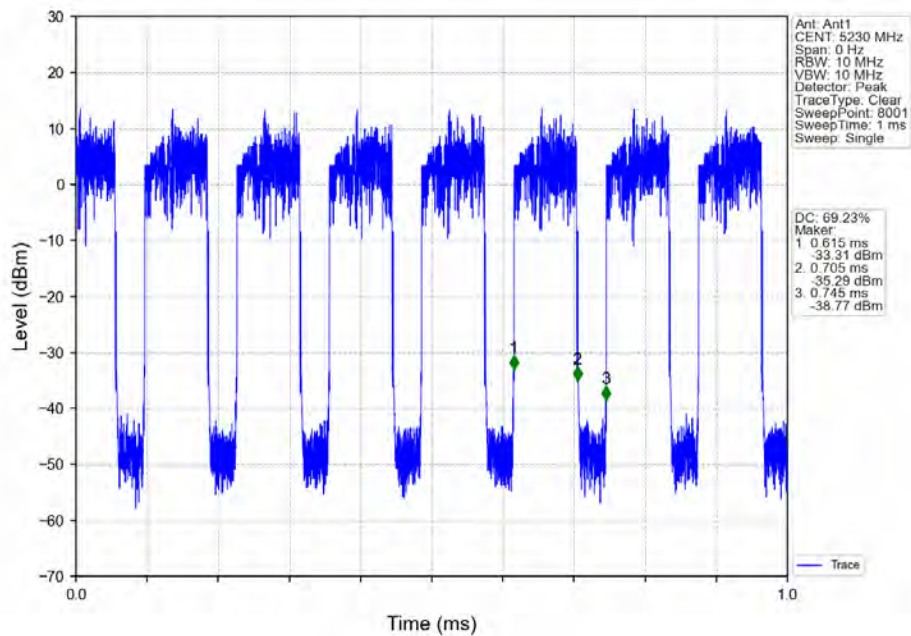
802.11ac(VHT40)_HCH_5230MHz_Ant1_NTNV
