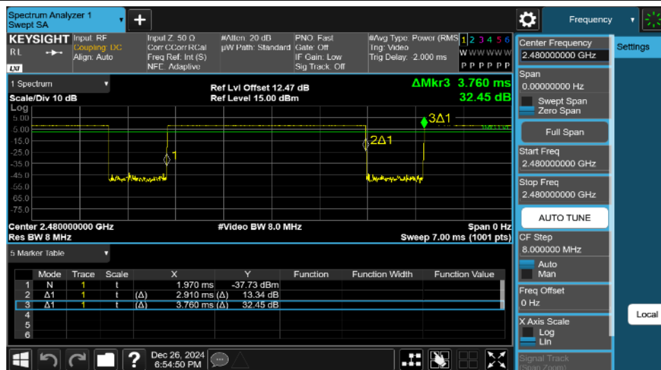
NTNV-DH5-Ant1-2480
