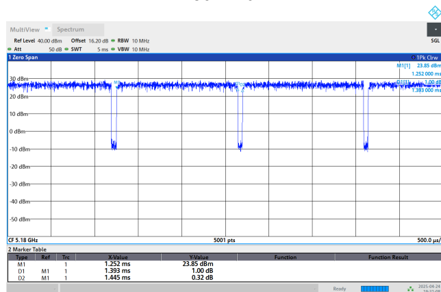
802.11a
