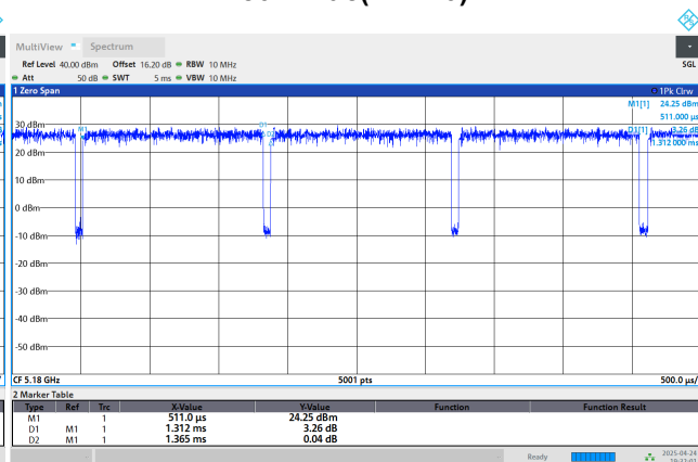
802.11ac(VHT20)
