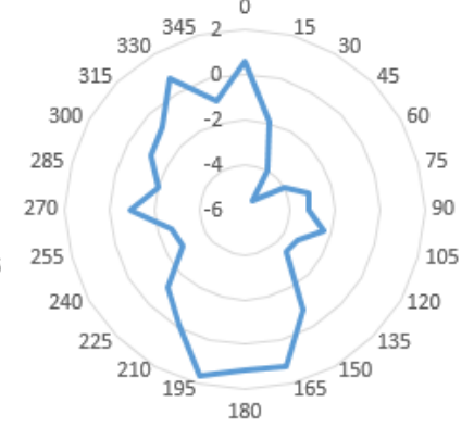
Theta=90°_5750MHz
