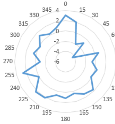
Theta=90°_5250MHz
