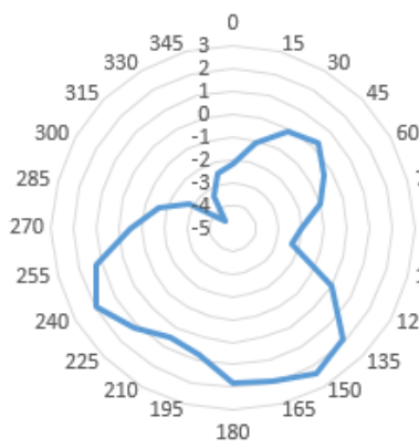
Theta=90°_2450MHz
