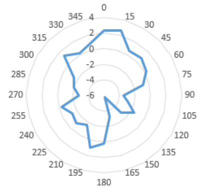
Theta=90°_5750MHz
