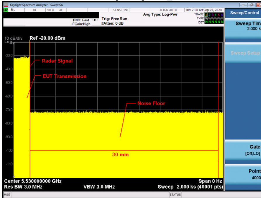
IEEE 802.11ax(VHT80) Mode_5530MHz
