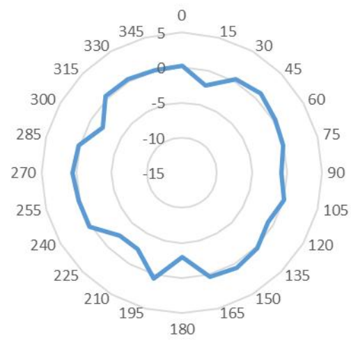
5250MHz
