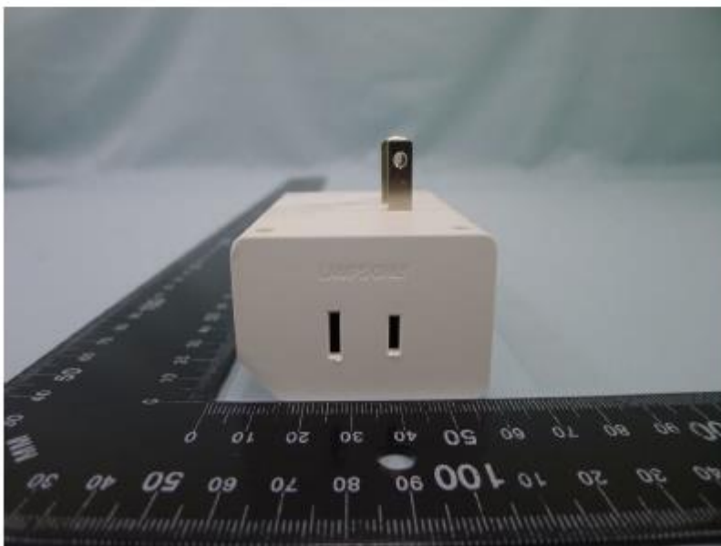
(6) EUT Photo
