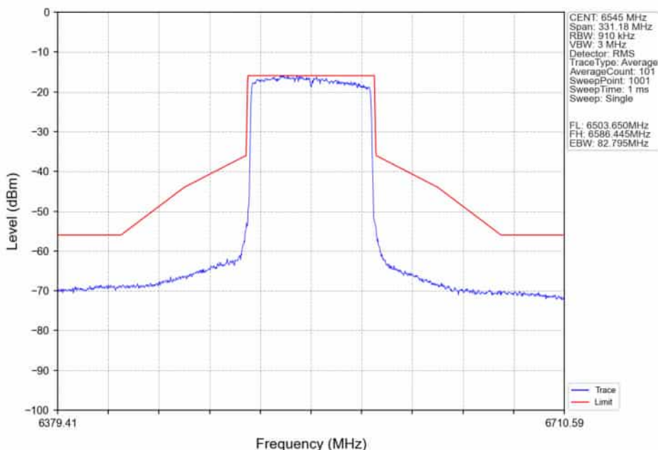
802.11ax(HEW80)_HCH_6545MHz_RU996_Left_Ant2_NTNV
