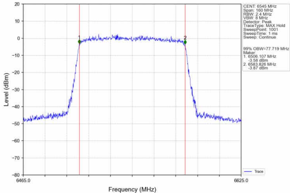
802.11ax(HEW80)_HCH_6545MHz_RU996_Left_Ant2_NTNV
