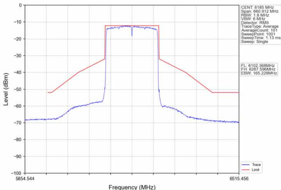
802.11ax(HEW160)_MCH_6185MHz_2xRU996_Left_Ant2_NTNV
