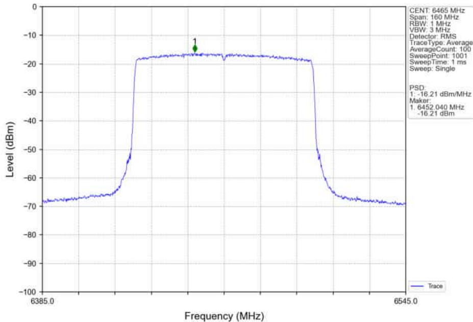
802.11ax(HEW80)_LCH_6465MHz_RU996_Left_MIMO_NTNV
