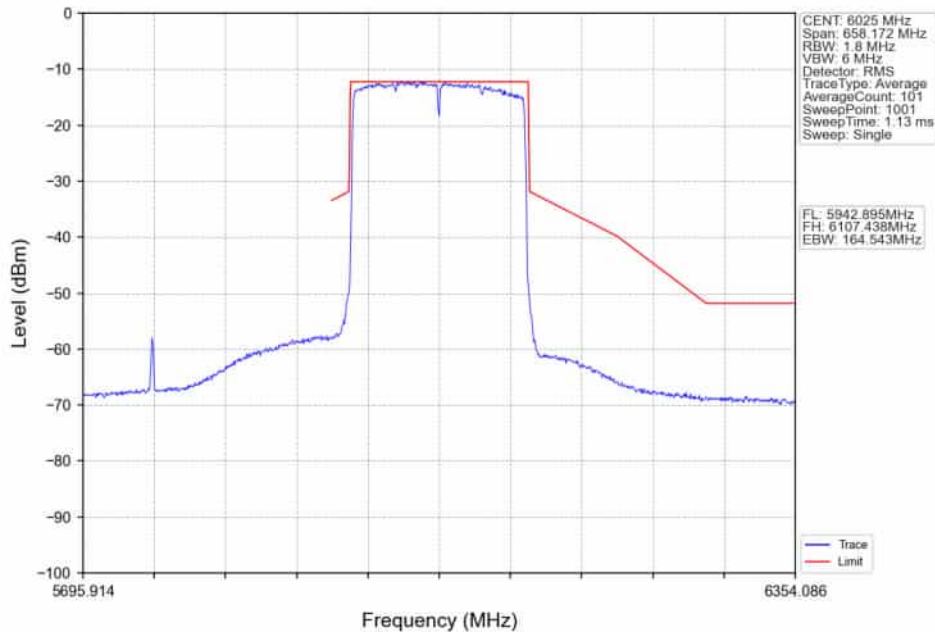
802.11ax(HEW160)_LCH_6025MHz_2xRU996_Left_Ant2_NTNV
