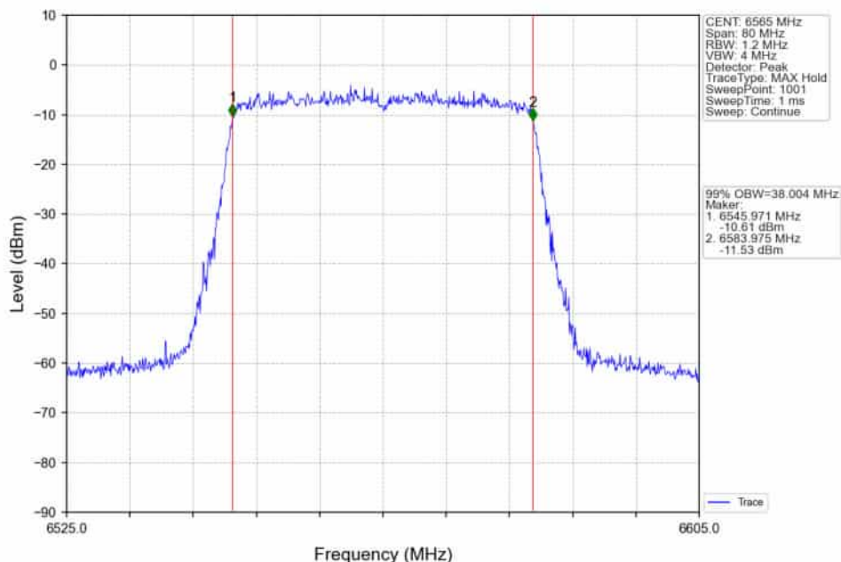
802.11ax(HEW40)_LCH_6565MHz_RU484_Left_Ant2_NTNV
