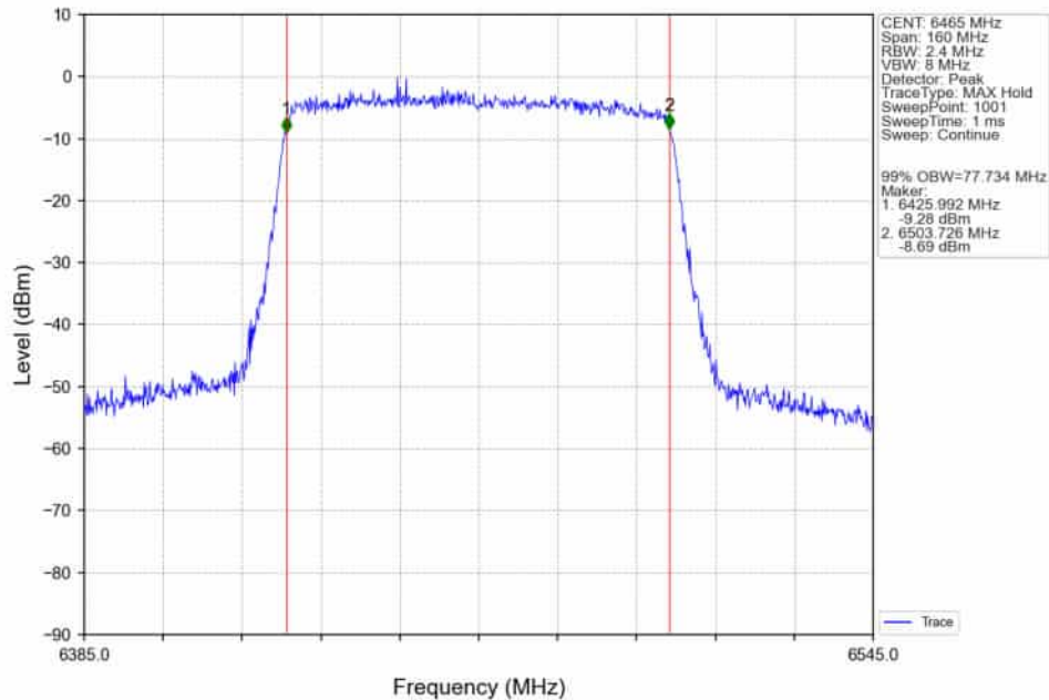
802.11ax(HEW80)_LCH_6465MHz_RU996_Left_Ant2_NTNV
