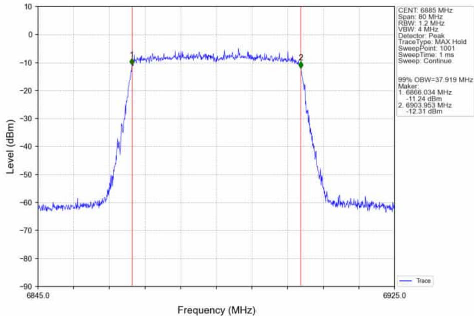
802.11ax(HEW40)_HCH_6885MHz_RU484_Left_Ant2_NTNV
