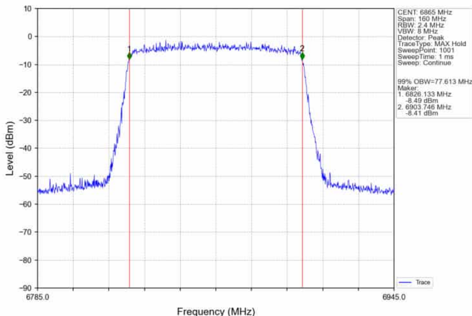
802.11ax(HEW80)_HCH_6865MHz_RU996_Left_Ant2_NTNV
