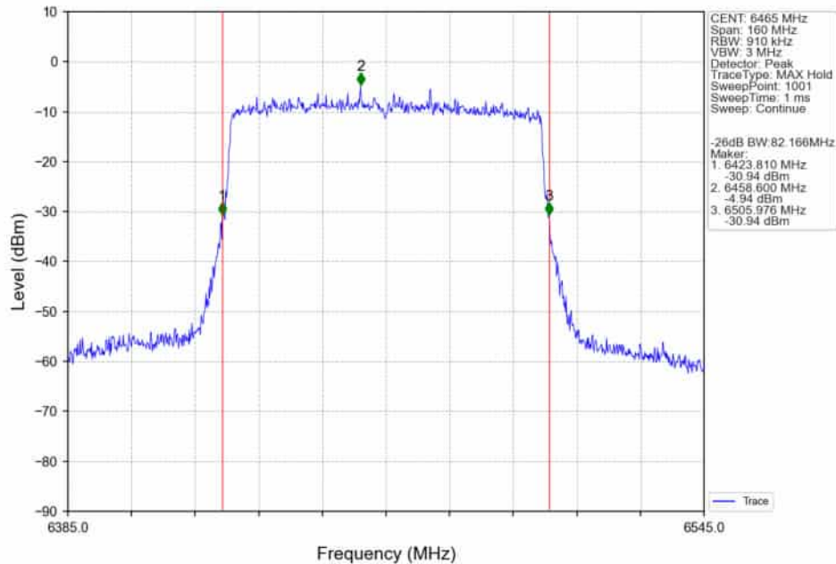
802.11ax(HEW80)_LCH_6465MHz_RU996_Left_Ant2_NTNV
