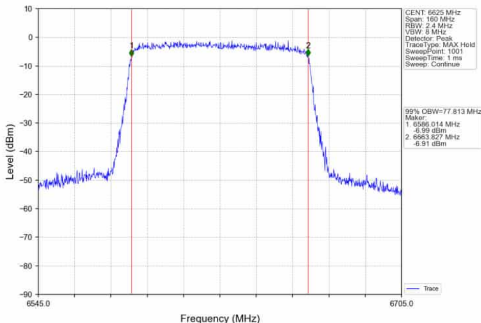
802.11ax(HEW80)_LCH_6625MHz_RU996_Left_Ant2_NTNV
