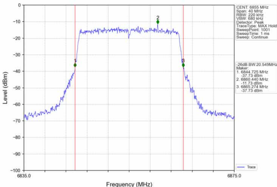
802.11ax(HEW20)_HCH_6855MHz_RU242_Left_Ant2_NTNV
