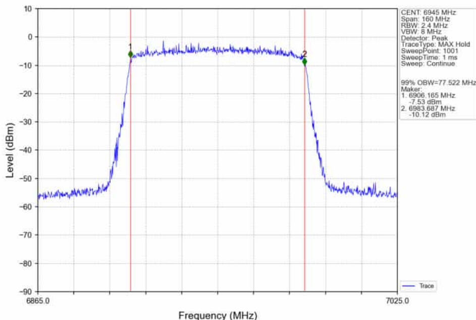
802.11ax(HEW80)_LCH_6945MHz_RU996_Left_Ant2_NTNV
