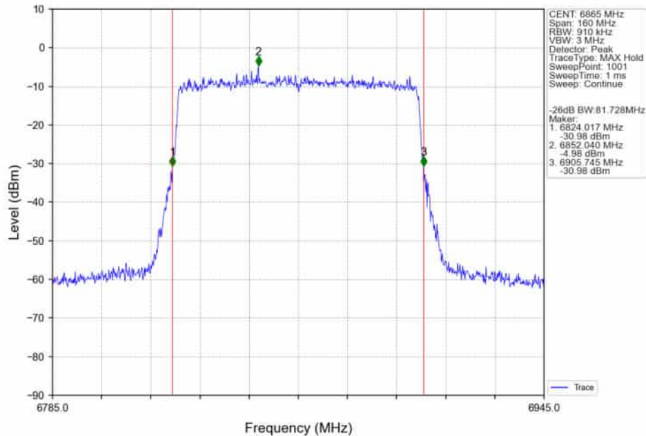
802.11ax(HEW80)_HCH_6865MHz_RU996_Left_Ant2_NTNV
