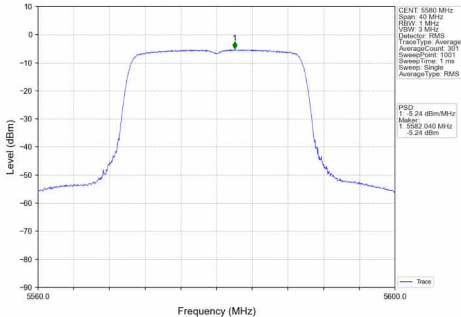
802.11ax(HE20)_MCH_5580MHz_RU242_Left_Ant1_NTNV
