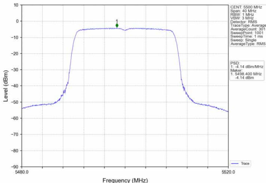
802.11ax(HE20)_LCH_5500MHz_RU242_Left_Ant2_NTNV
