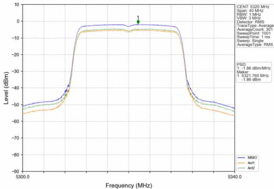
802.11ax(HE20)_HCH_5320MHz_RU242_Left_MIMO_NTNV
