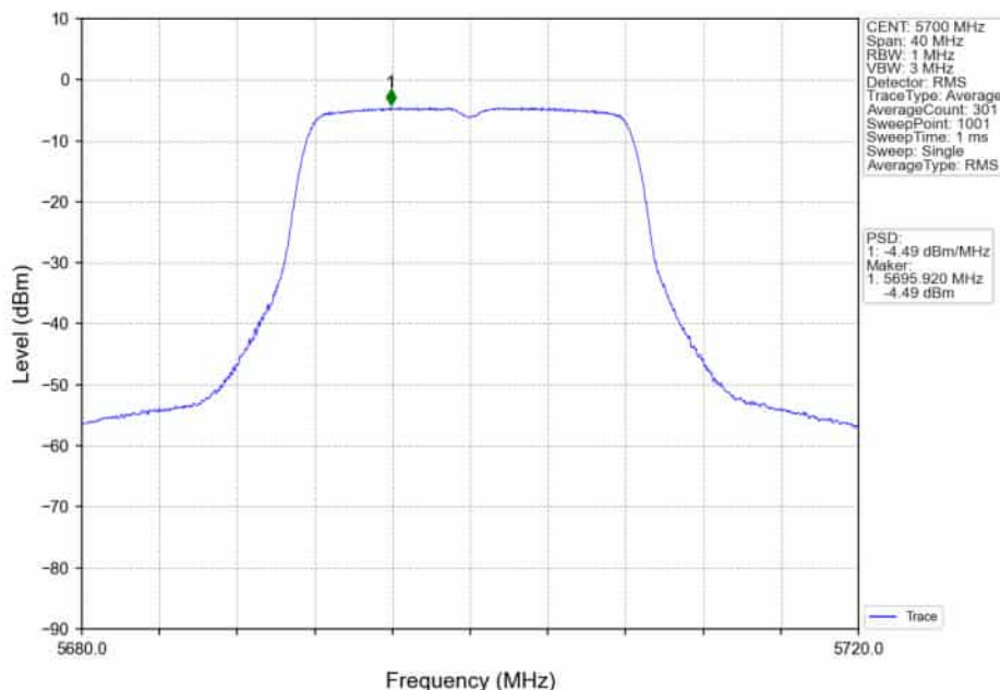
802.11a_HCH_5700MHz_Ant2_NTNV
