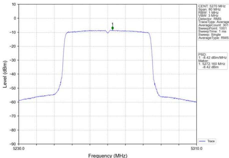
802.11ax(HE40)_LCH_5270MHz_RU484_Left_Ant1_NTNV
