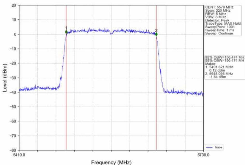
802.11ax(HE160)_MCH_5570MHz_2xRU996_Left_Ant2_NTNV
