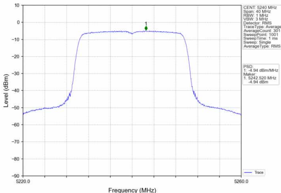
802.11ax(HE20)_HCH_5240MHz_RU242_Left_Ant2_NTNV
