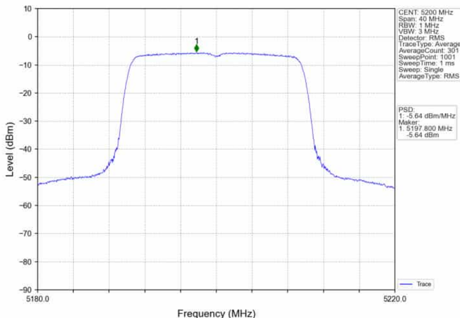
802.11ax(HE20)_MCH_5200MHz_RU242_Left_Ant1_NTNV
