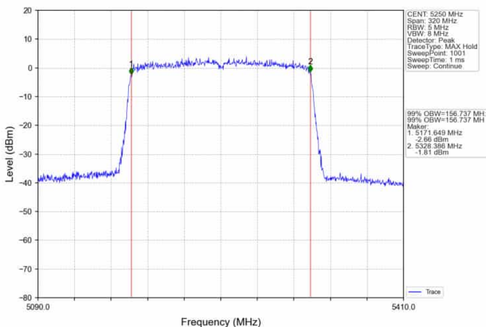
802.11ax(HE160)_MCH_5250MHz_2xRU996_Left_Ant2_NTNV
