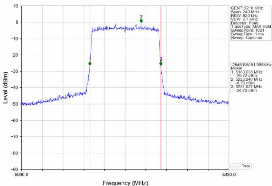
802.11ax(HE80)_MCH_5210MHz_RU996_Left_Ant2_NTNV
