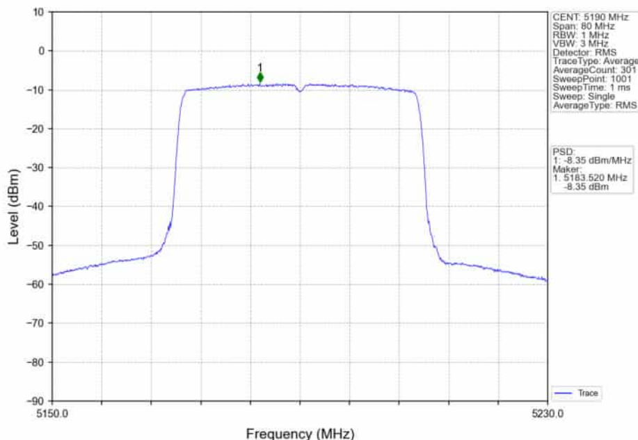
802.11ax(HE40)_LCH_5190MHz_RU484_Left_Ant1_NTNV
