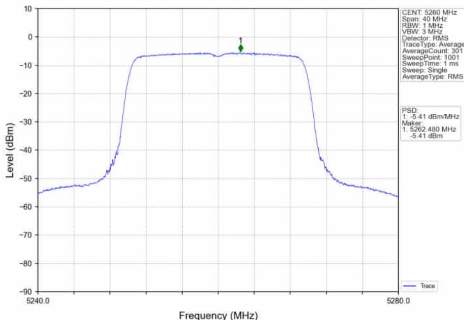
802.11ax(HE20)_LCH_5260MHz_RU242_Left_Ant1_NTNV
