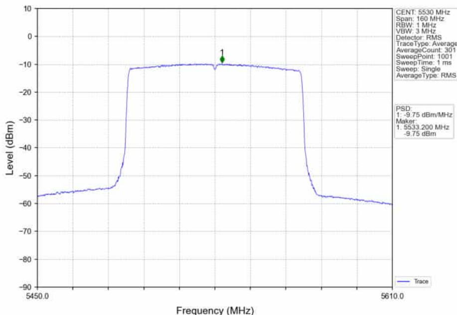
802.11ax(HE80)_LCH_5530MHz_RU996_Left_Ant2_NTNV
