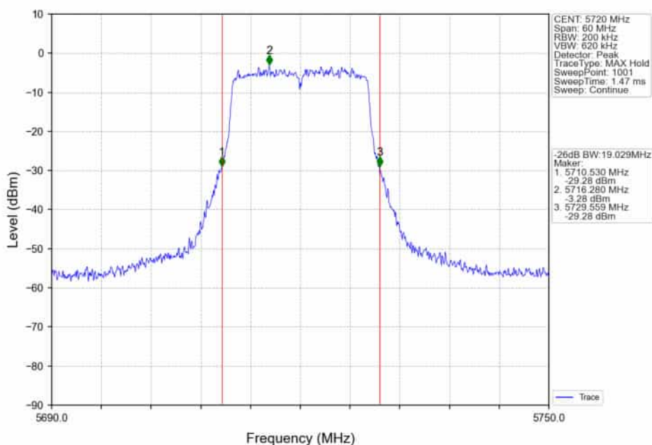
802.11a_HCH_5720MHz_Ant2_NTNV
