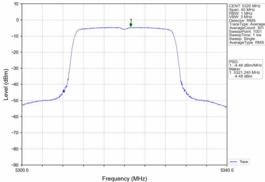
802.11ax(HE20)_HCH_5320MHz_RU242_Left_Ant2_NTNV
