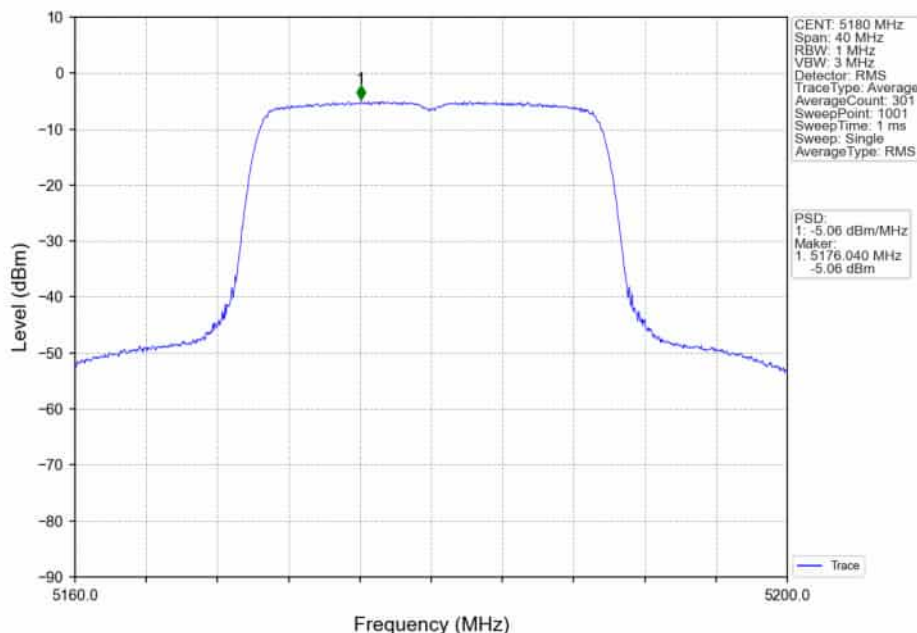
802.11ax(HE20)_LCH_5180MHz_RU242_Left_Ant2_NTNV
