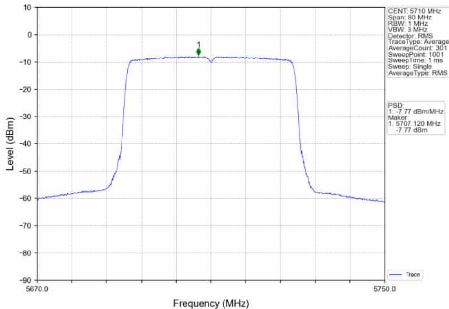
802.11ax(HE40)_HCH_5710MHz_RU484_Left_Ant2_NTNV
