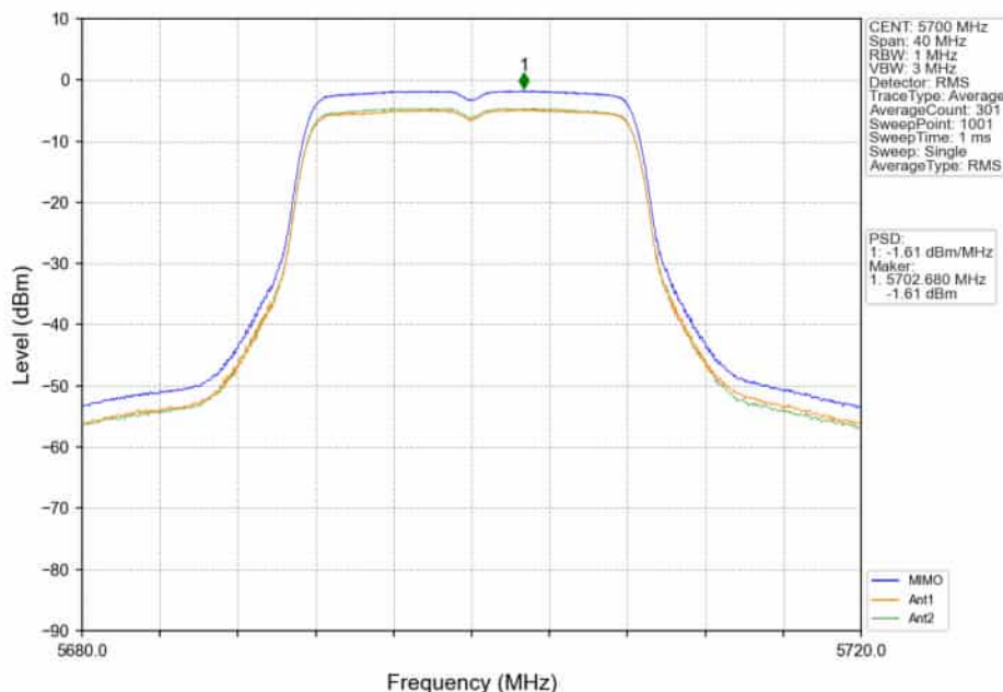
802.11a_HCH_5700MHz_MIMO_NTNV
