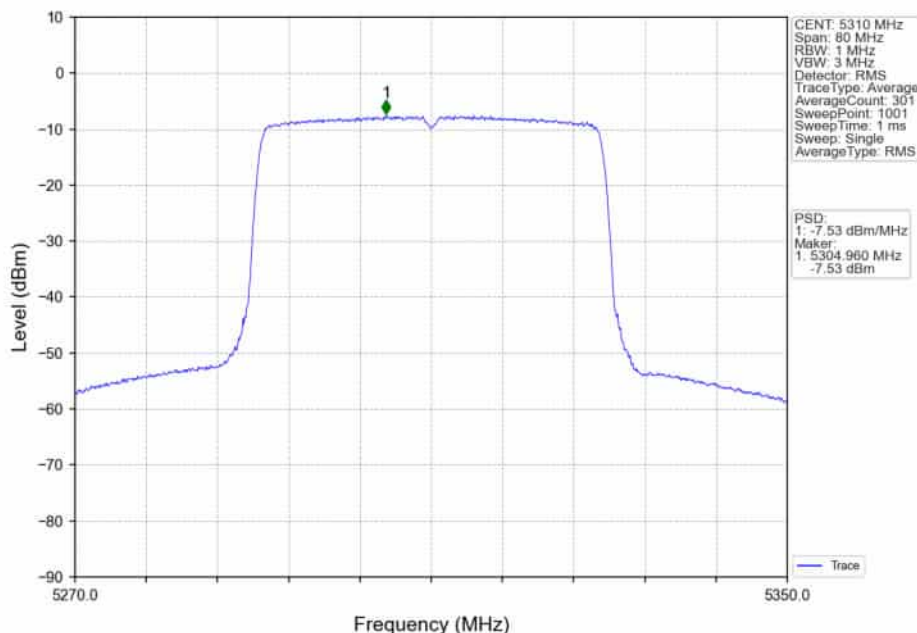
802.11ax(HE40)_HCH_5310MHz_RU484_Left_Ant2_NTNV
