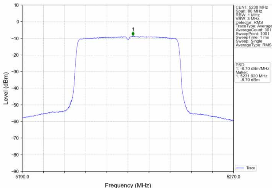
802.11ax(HE40)_HCH_5230MHz_RU484_Left_Ant1_NTNV
