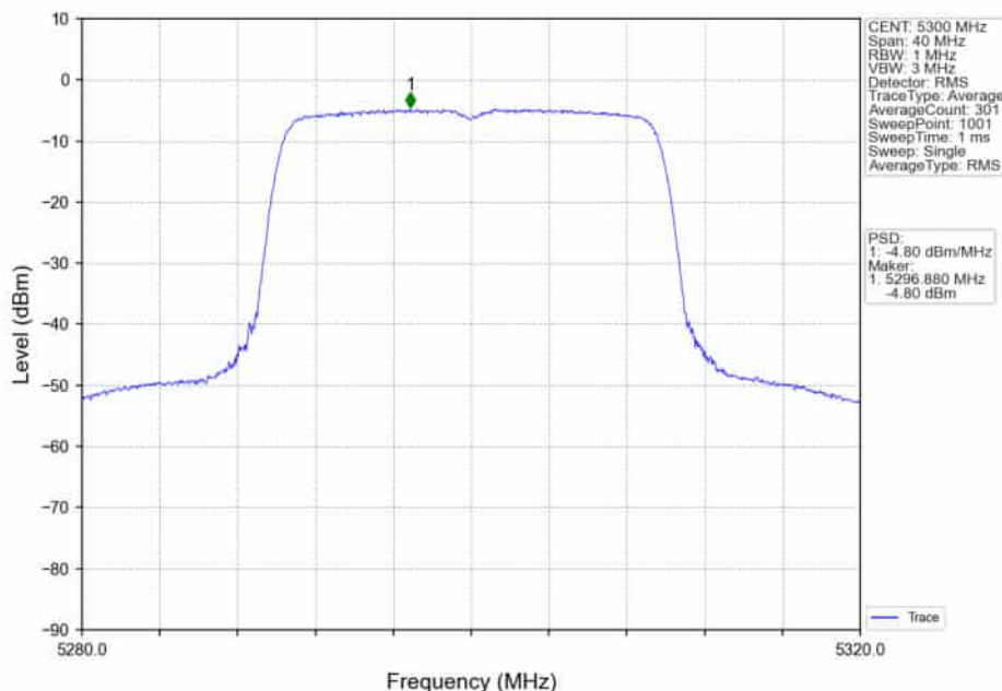
802.11ax(HE20)_MCH_5300MHz_RU242_Left_Ant2_NTNV
