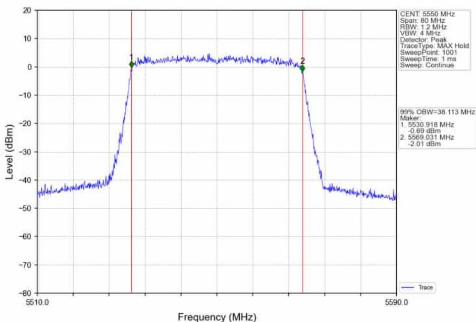
802.11ax(HE40)_MCH_5550MHz_RU484_Left_Ant2_NTNV
