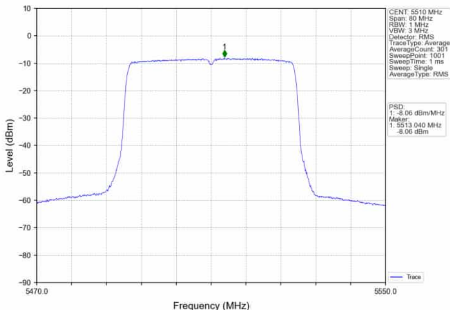
802.11ax(HE40)_LCH_5510MHz_RU484_Left_Ant1_NTNV
