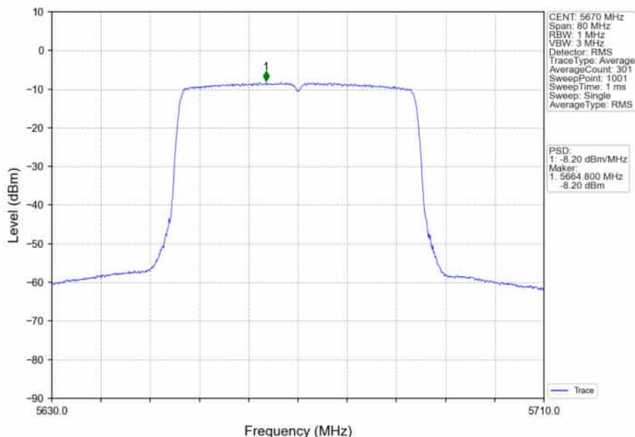
802.11ax(HE40)_HCH_5670MHz_RU484_Left_Ant2_NTNV
