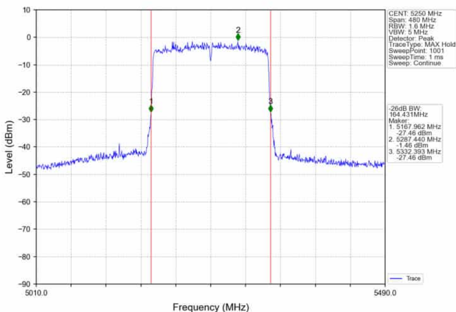
802.11ax(HE160)_MCH_5250MHz_2xRU996_Left_Ant2_NTNV
