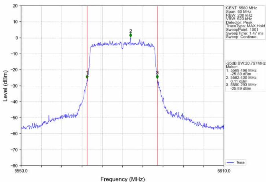
802.11ax(HE20)_MCH_5580MHz_RU242_Left_Ant2_NTNV
