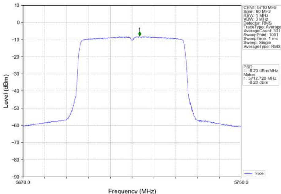
802.11ax(HE40)_HCH_5710MHz_RU484_Left_Ant1_NTNV
