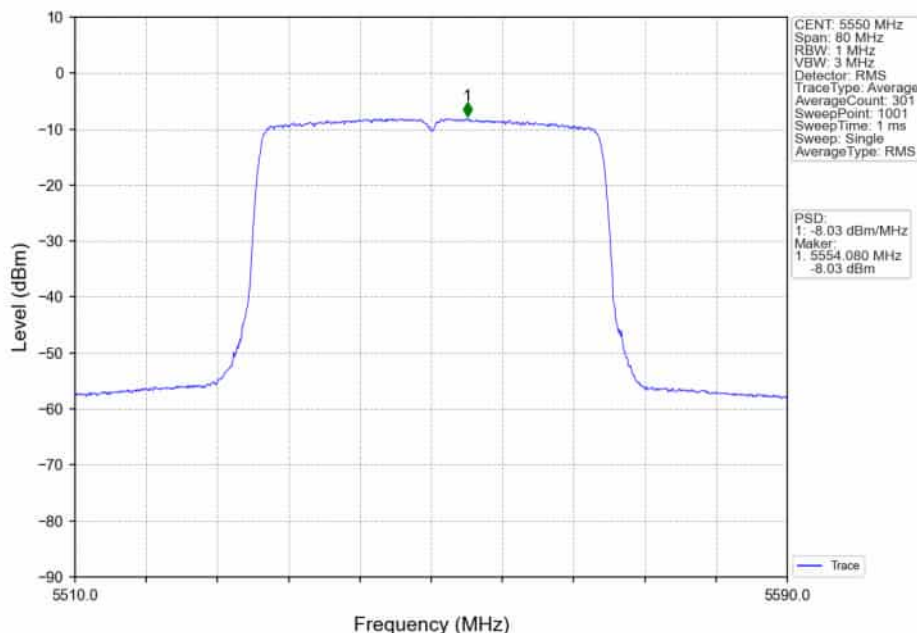
802.11ax(HE40)_MCH_5550MHz_RU484_Left_Ant1_NTNV
