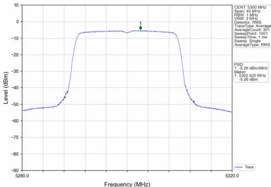
802.11ax(HE20)_MCH_5300MHz_RU242_Left_Ant1_NTNV
