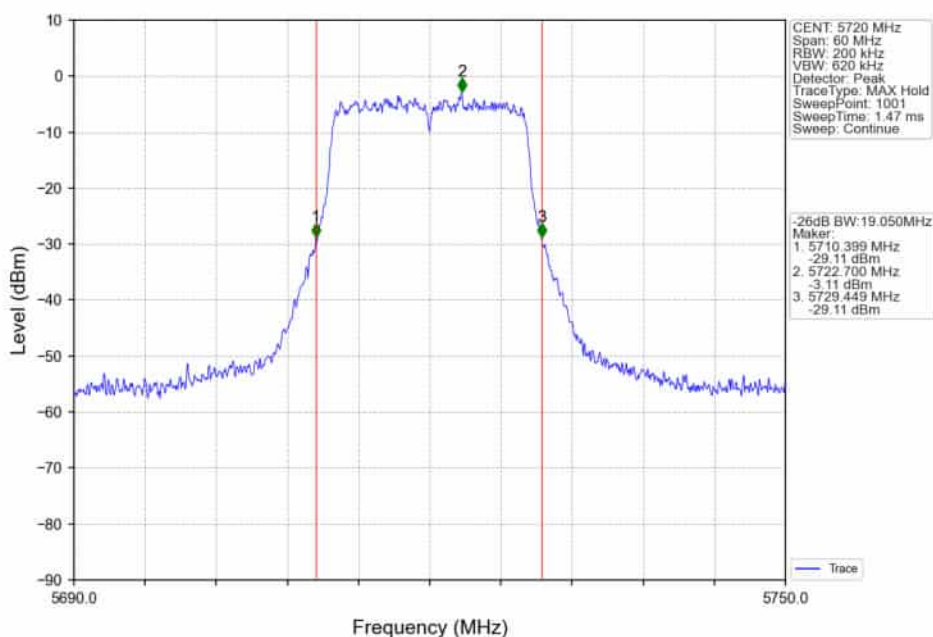
802.11a_HCH_5720MHz_Ant1_NTNV
