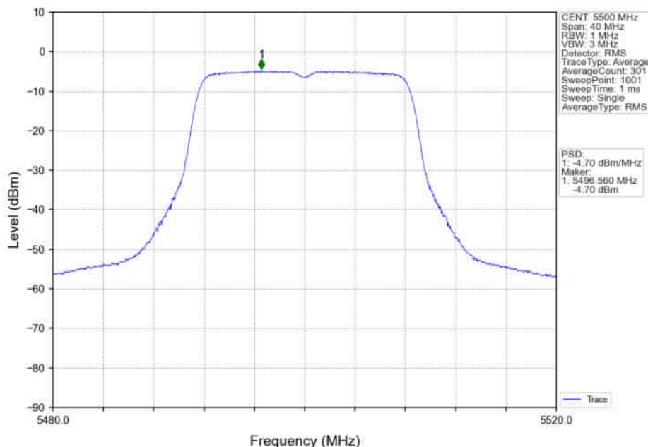
802.11a_LCH_5500MHz_Ant1_NTNV
