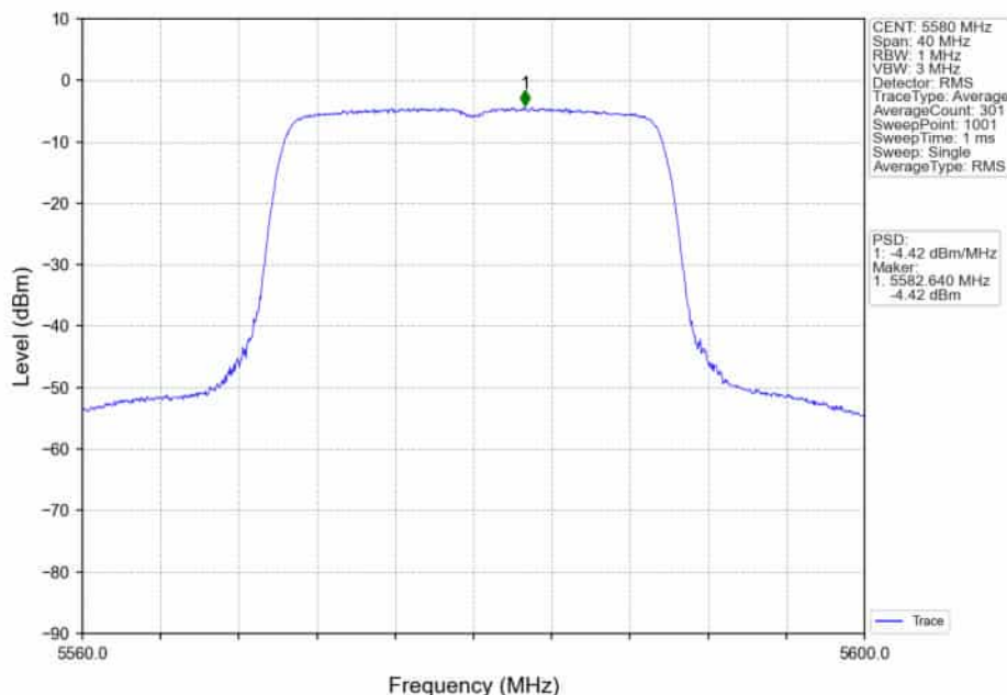
802.11ax(HE20)_MCH_5580MHz_RU242_Left_Ant2_NTNV
