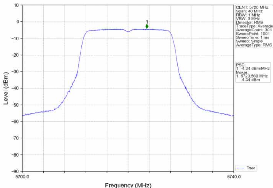
802.11a_HCH_5720MHz_Ant2_NTNV
