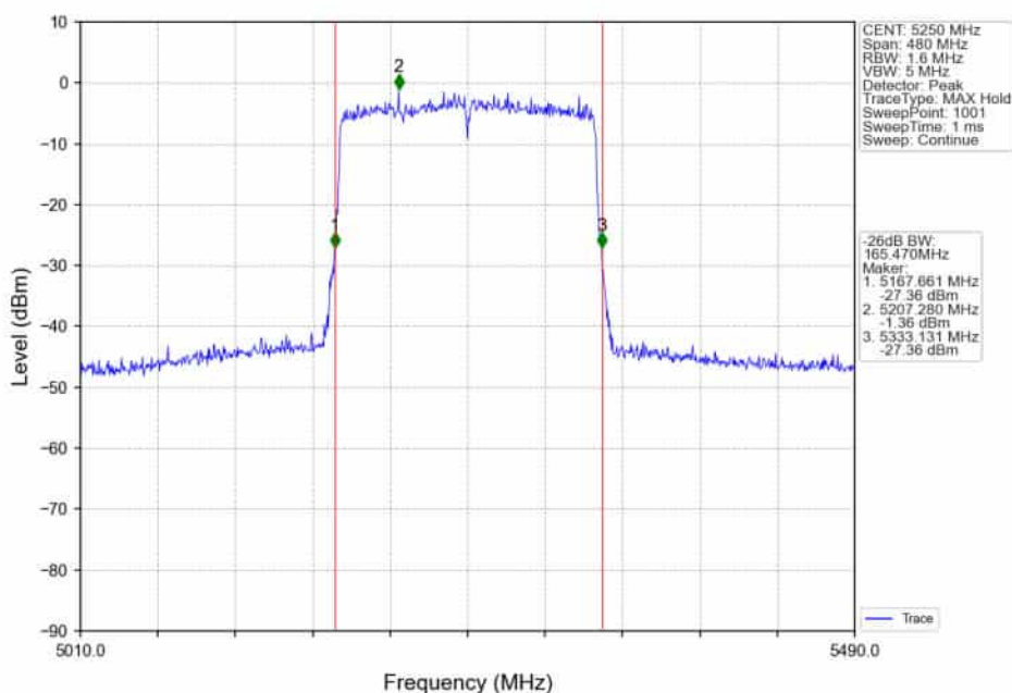
802.11ax(HE160)_MCH_5250MHz_2xRU996_Left_Ant1_NTNV
