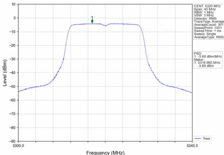
802.11a_HCH_5320MHz_Ant2_NTNV
