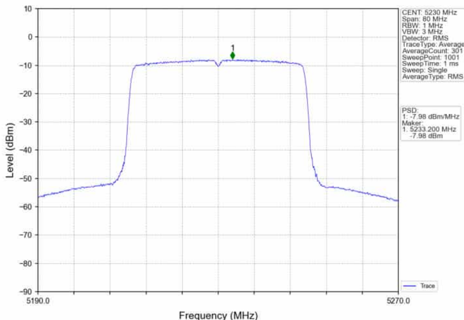
802.11ax(HE40)_HCH_5230MHz_RU484_Left_Ant2_NTNV
