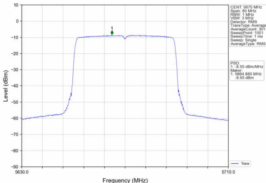
802.11ax(HE40)_HCH_5670MHz_RU484_Left_Ant1_NTNV
