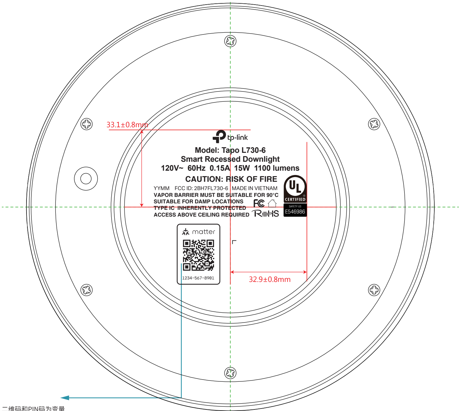
结构图
