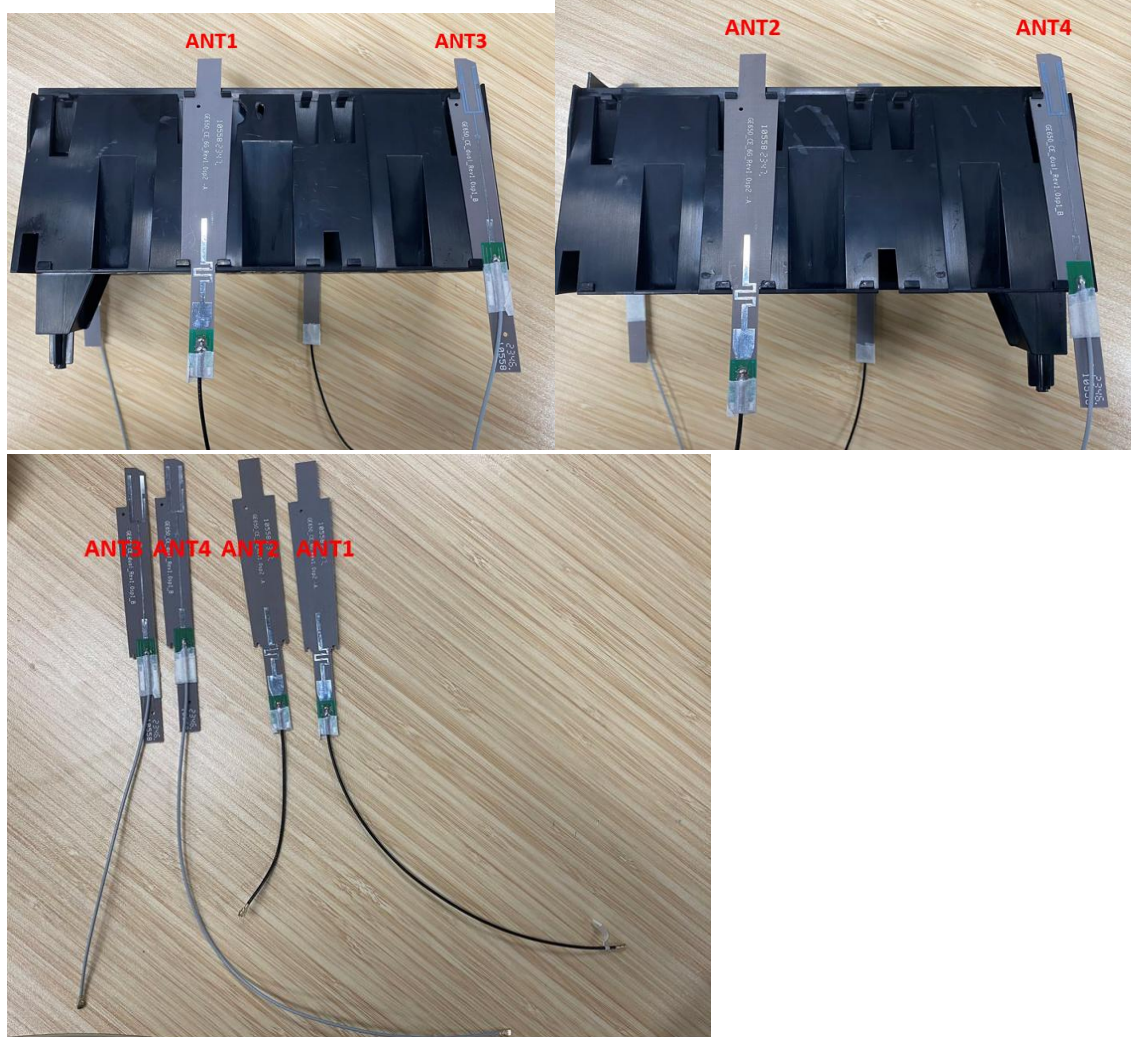
Archer GE550
