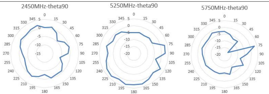
Ant4
