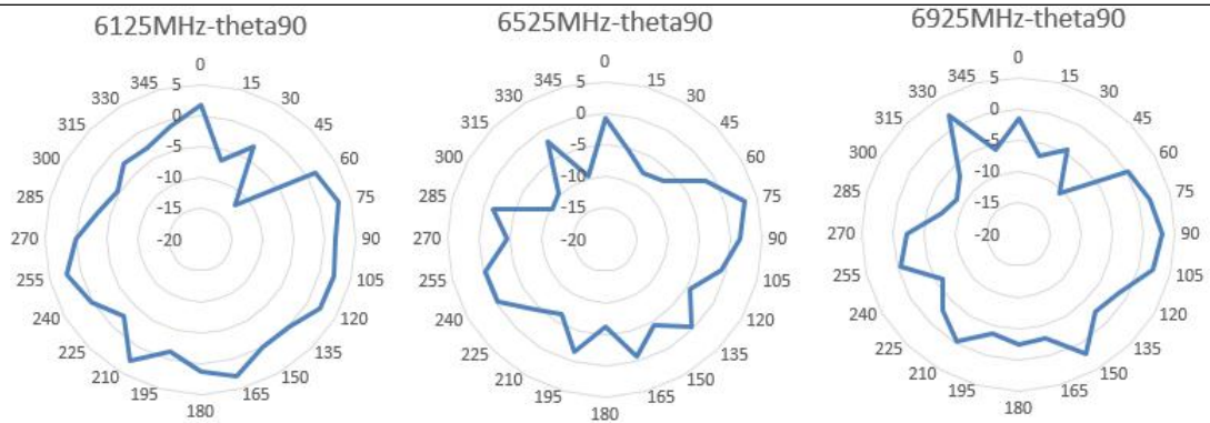
Ant1
