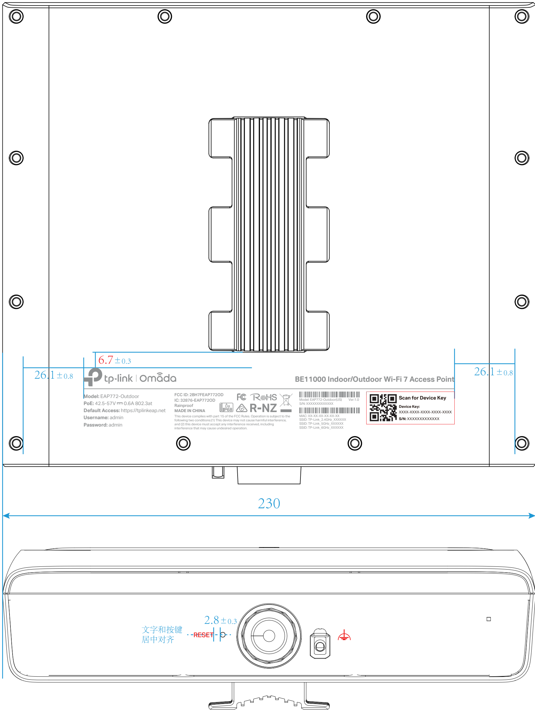
尺寸图
