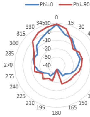
5250MHz_Phi=0&Phi=90
