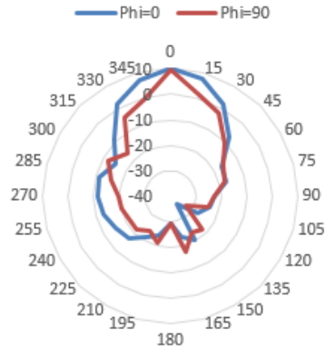
5750MHz_Phi=0&Phi=90
