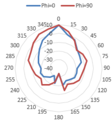
5750MHz_Phi=0&Phi=90
