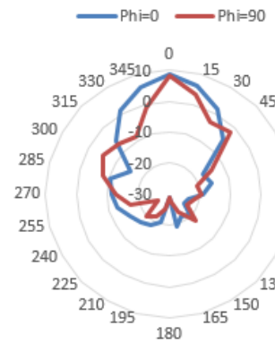
5250MHz_Phi=0&Phi=90
