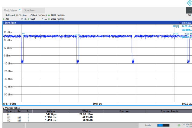
IEEE 802.11a
