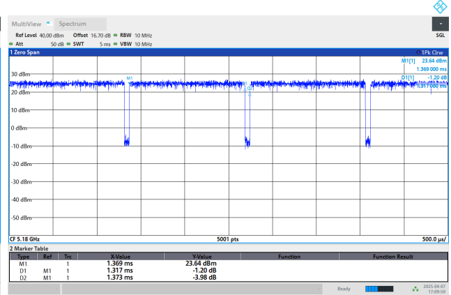
IEEE 802.11ac(VHT20)
