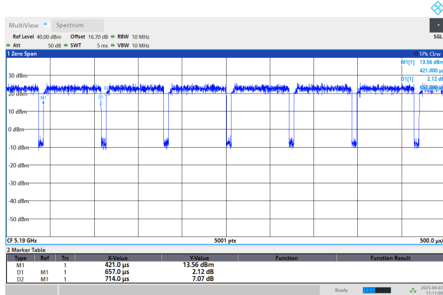
IEEE 802.11ac(VHT40)
