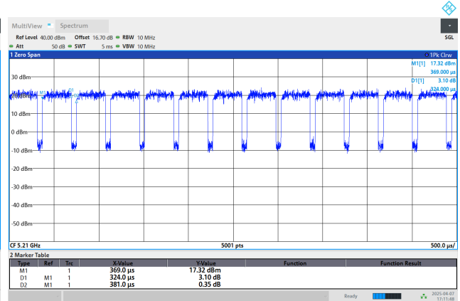
IEEE 802.11ac(VHT80)
