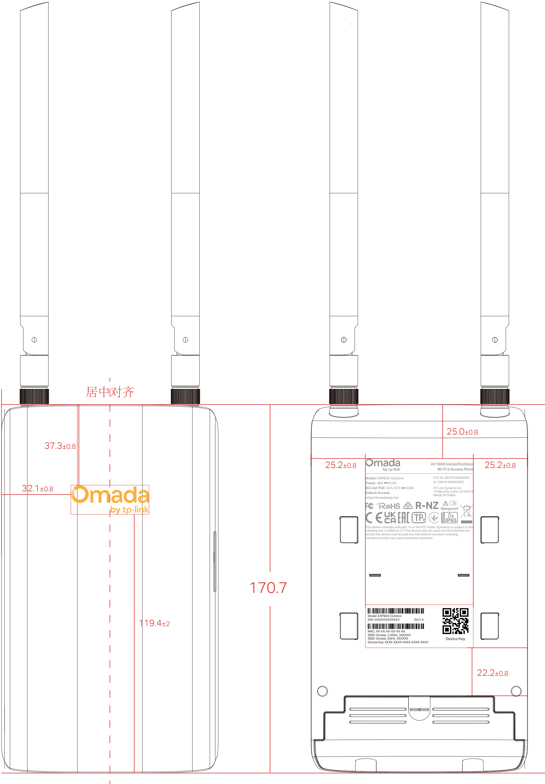
尺寸图
