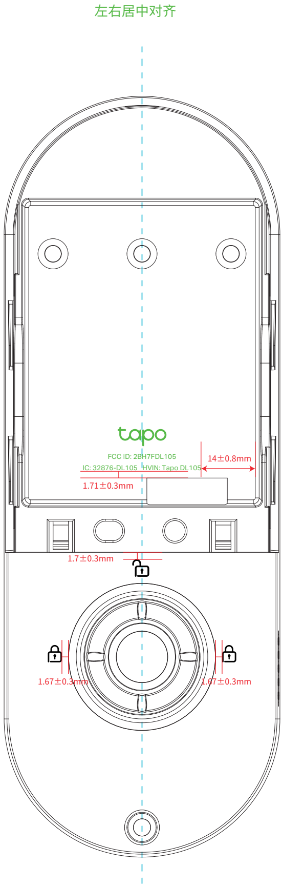
尺寸图
